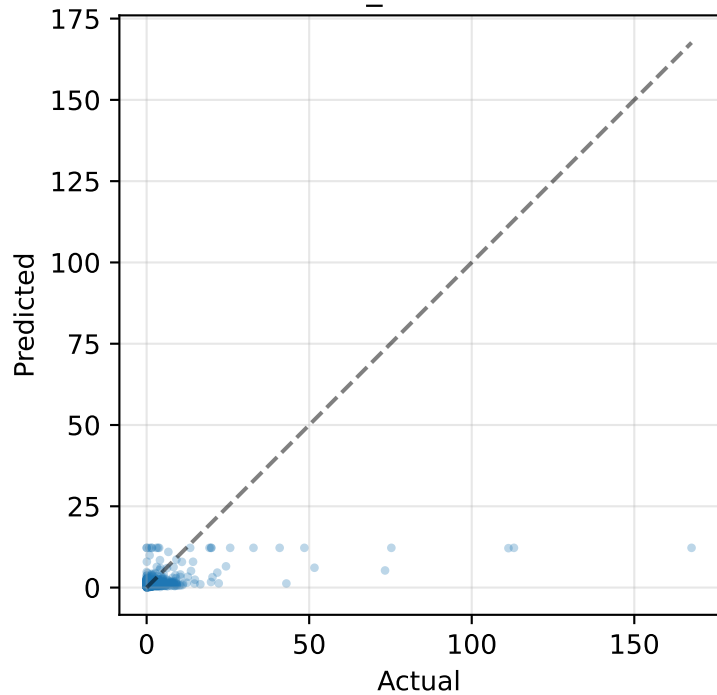
DNN_HAR+SVD
