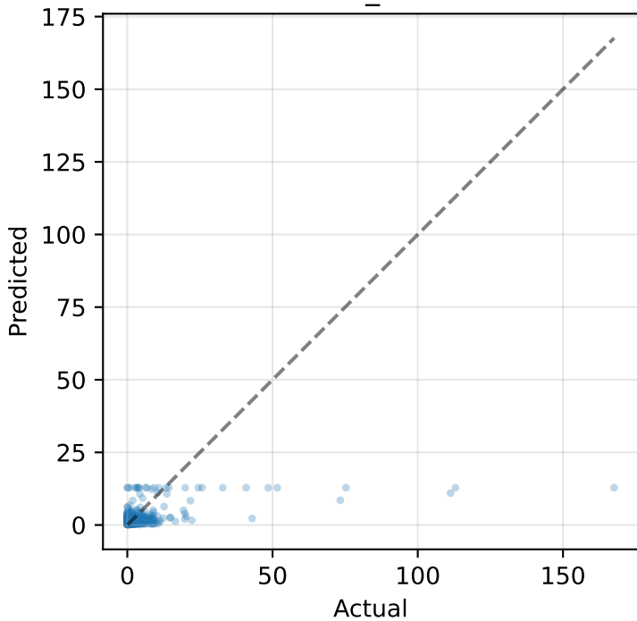
DNN_HAR
