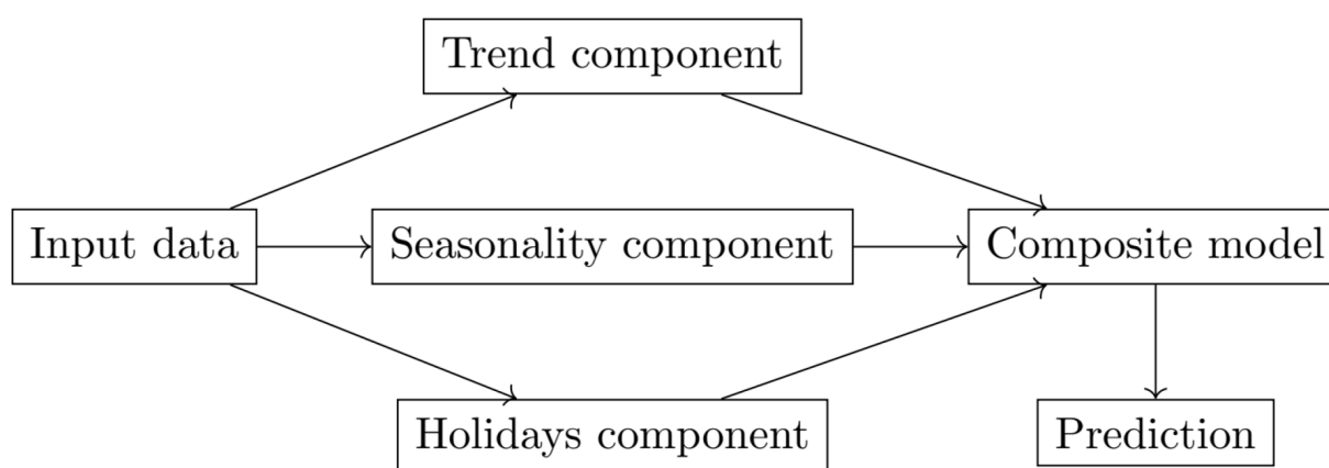
Figure 10: Principe Prophet: la prévision combine tendance et saisonnalités. Ce modèle complète le LSTM en donnant une lecture plus stable du comportement attendu.
