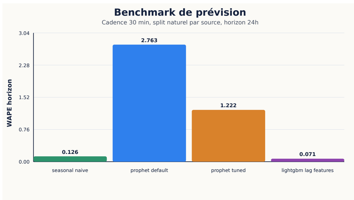
Figure 9: Comparaison WAPE sur horizon 24h. LightGBM obtient la meilleure précision brute sur ce jeu synthétique, tandis que Prophet reste le modèle le plus explicable pour raconter tendance et saisonnalité.
