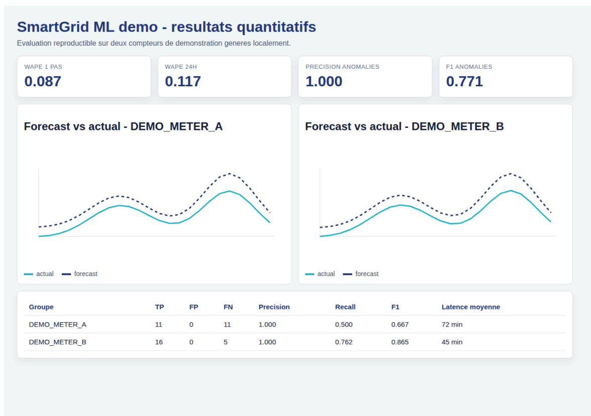
Figure 14: Synthèse locale des métriques ML: WAPE, précision, F1 et comparaison entre consommation réelle et prévue.
