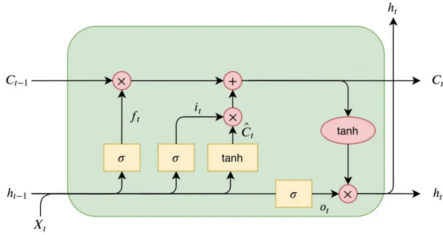
Figure 11: Architecture LSTM: les portes contrôlent la mémoire, l'oubli et la sortie. Cette structure reste utile pour une baseline séquentielle non supervisée.
