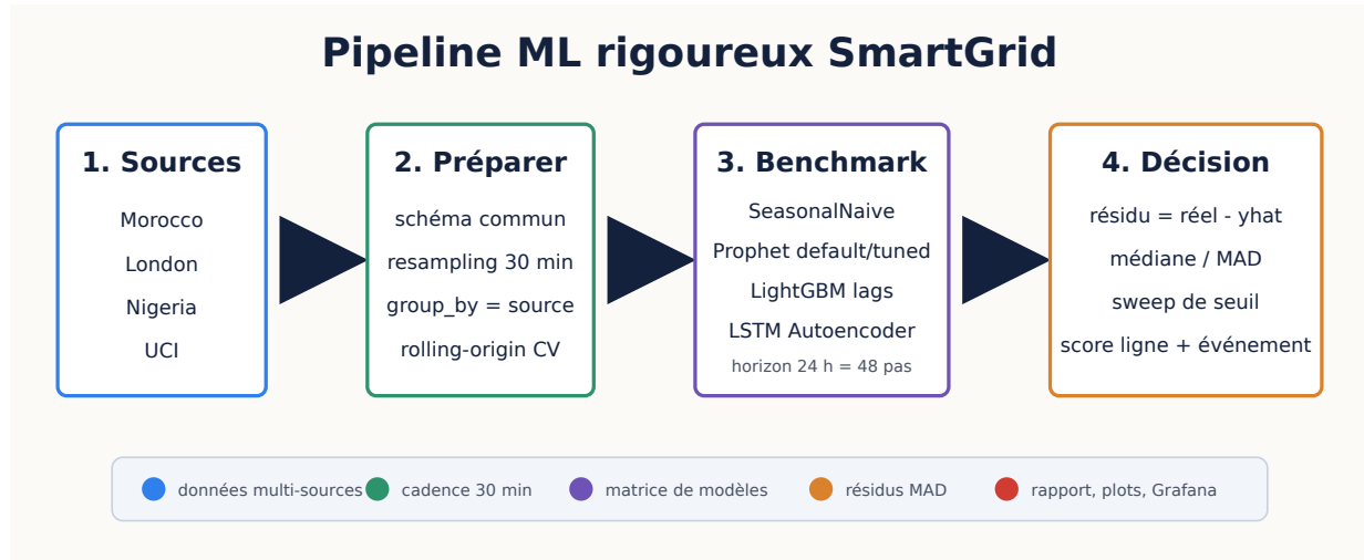
Figure 8: Pipeline ML retenu: sources de données, prétraitement à 30 minutes, benchmark de prévision, calcul du résidu, sélection du seuil MAD et restitution des anomalies dans Grafana.
