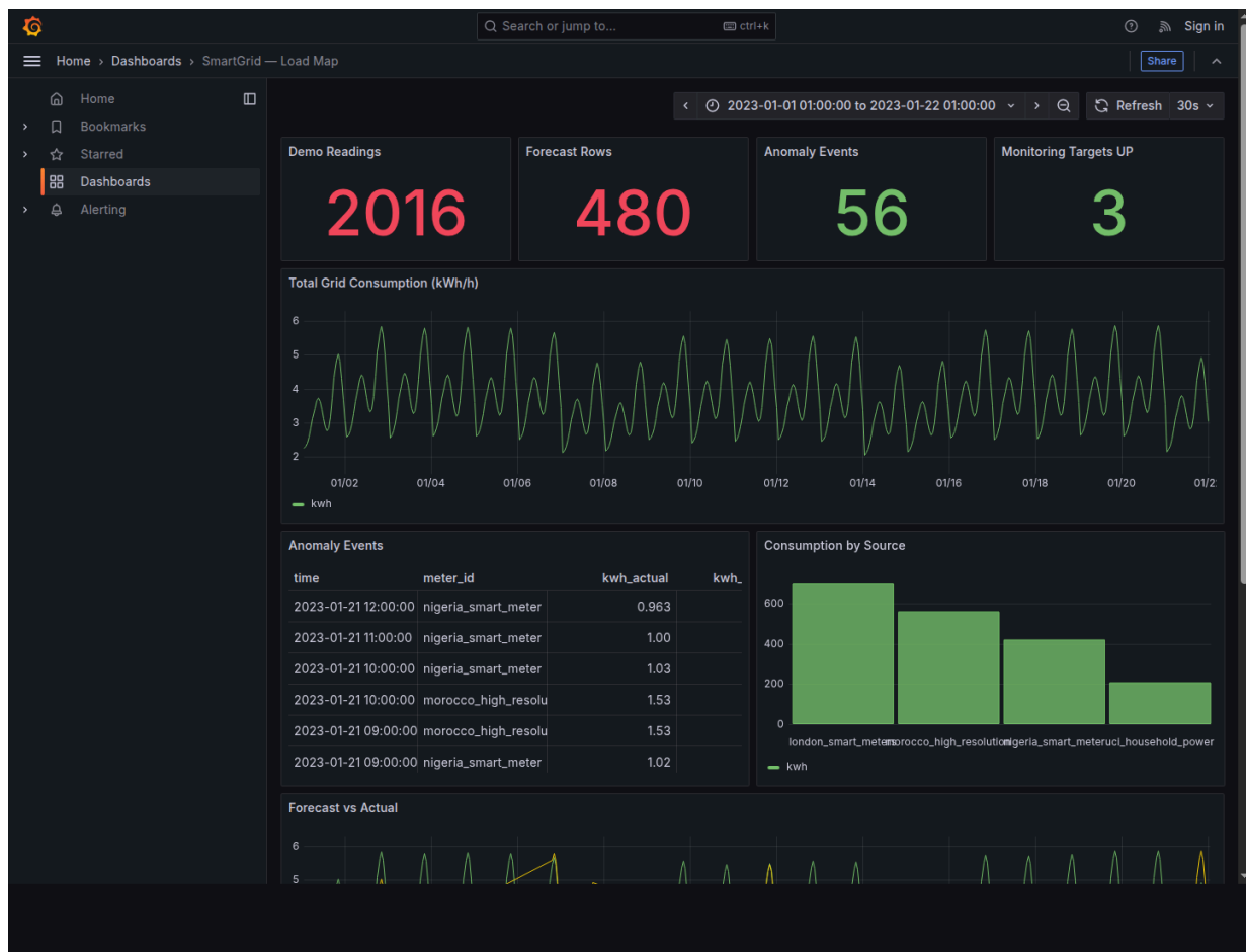
Figure 16: Grafana: dashboard SmartGrid peuplé avec lectures, prévisions, anomalies, consommation par source et indicateur de monitoring.
