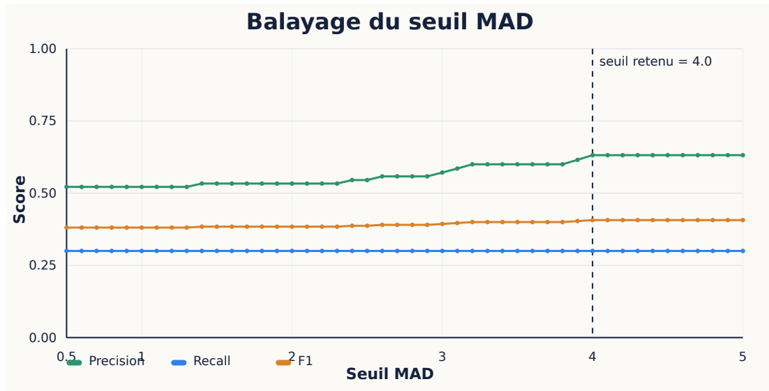
Figure 12: Balayage du seuil MAD sur les résidus LightGBM. Le seuil 4.0 est retenu comme point de fonctionnement pour préserver une précision raisonnable tout en gardant des alertes exploitables.
