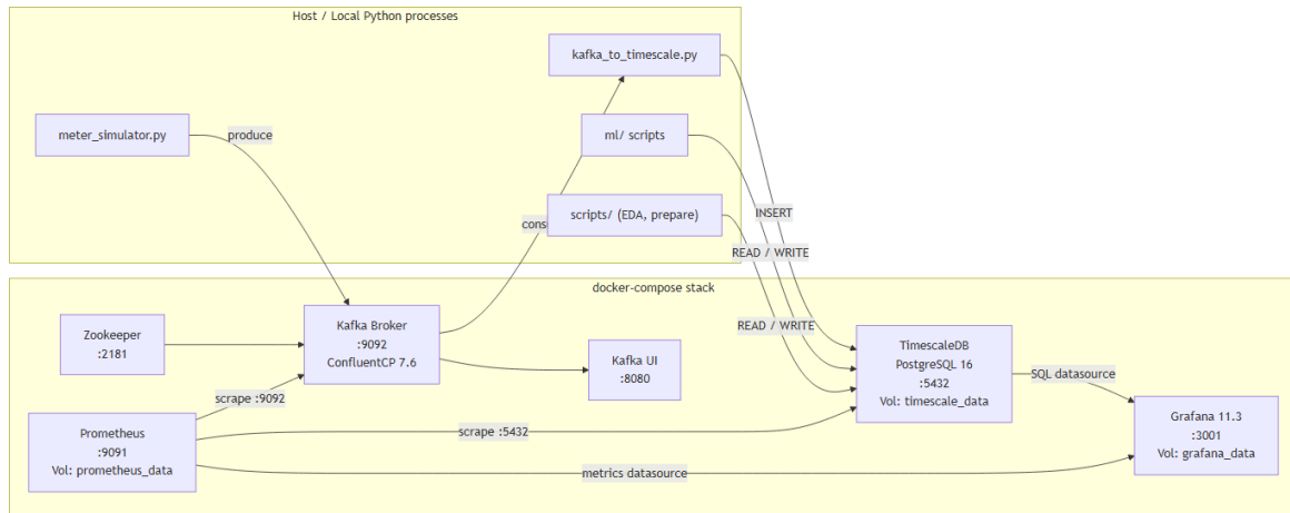
Figure 15: Topologie Docker Compose: Kafka pour l'ingestion, TimescaleDB pour les séries temporelles, Grafana pour la visualisation et Prometheus pour la supervision technique.
