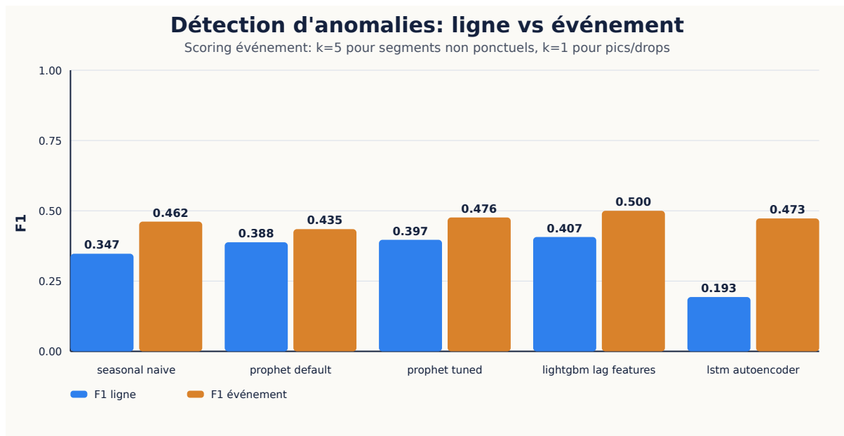
Figure 13: Comparaison F1 ligne vs F1 événement. Le scoring événement pénalise moins les micro-fluctuations isolées, mais révèle clairement que les anomalies contextuelles 02:00/14:00 et les drifts graduels restent difficiles pour un simple résidu MAD.
