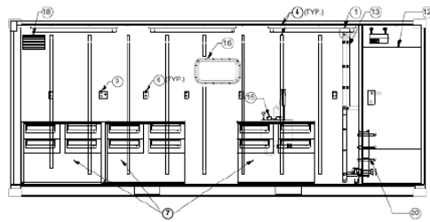
SECTION D-D
