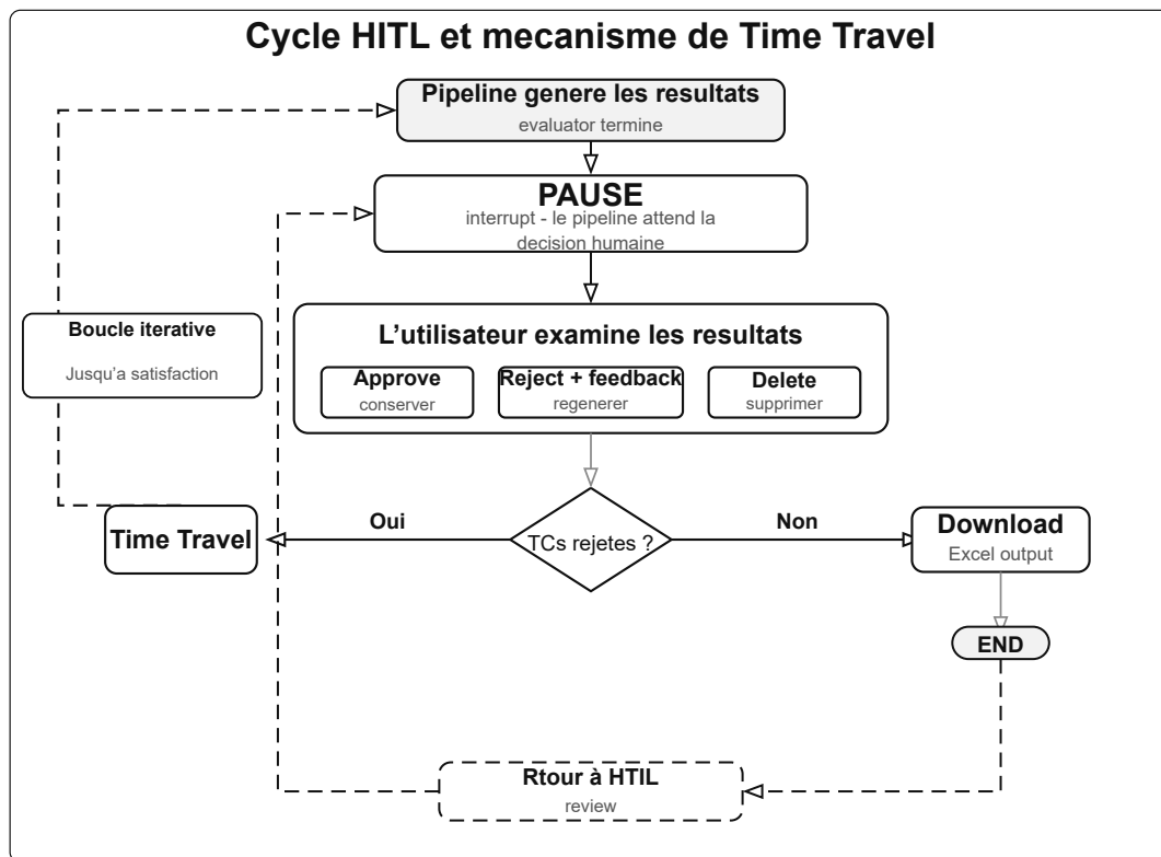
Figure 22: Cycle HITL et mécanisme de Time Travel
