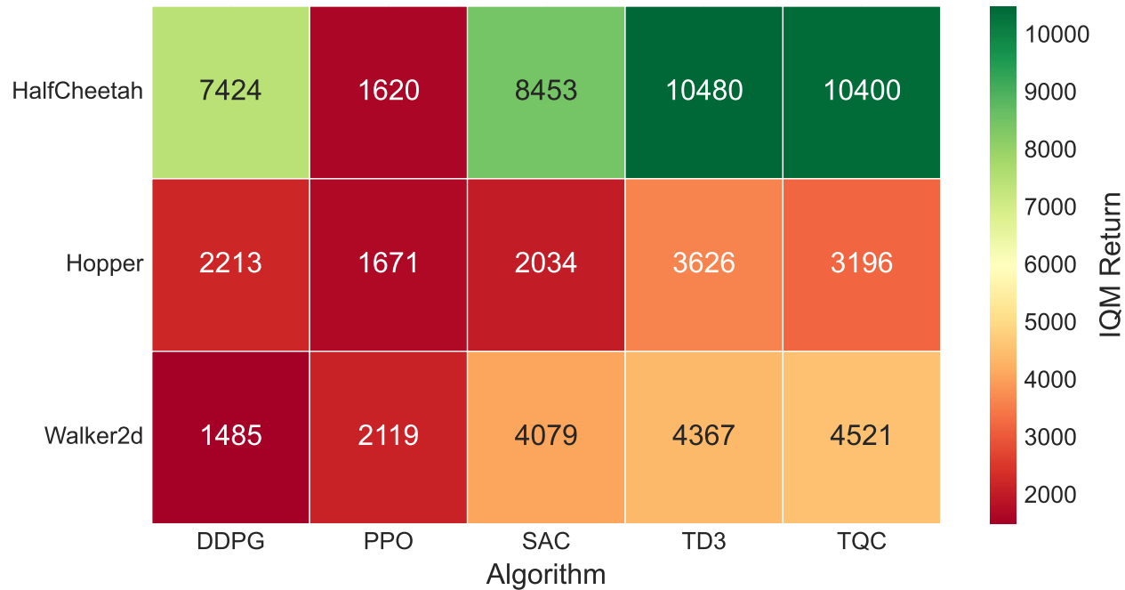
IQM Returns — Default 1M
