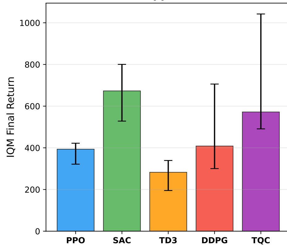
Hopper-v5
