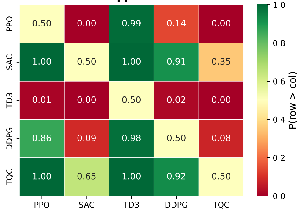
Hopper-v5
