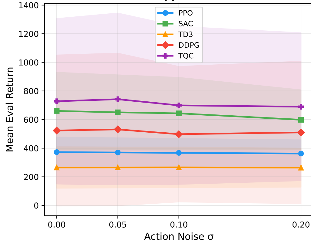
Hopper-v5
