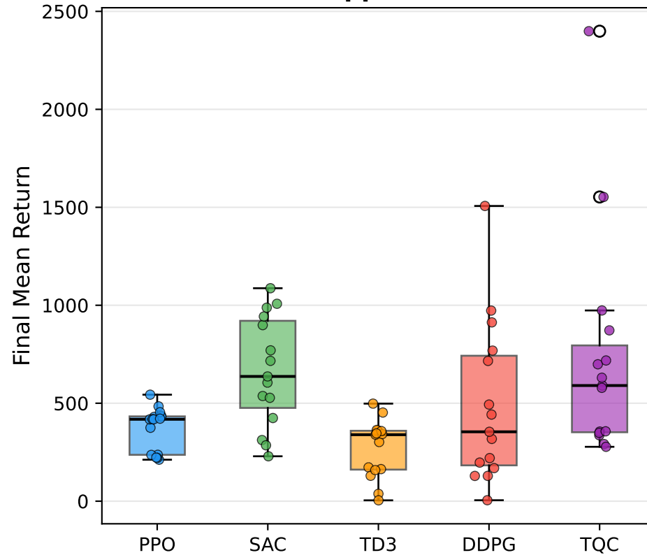
Hopper-v5
