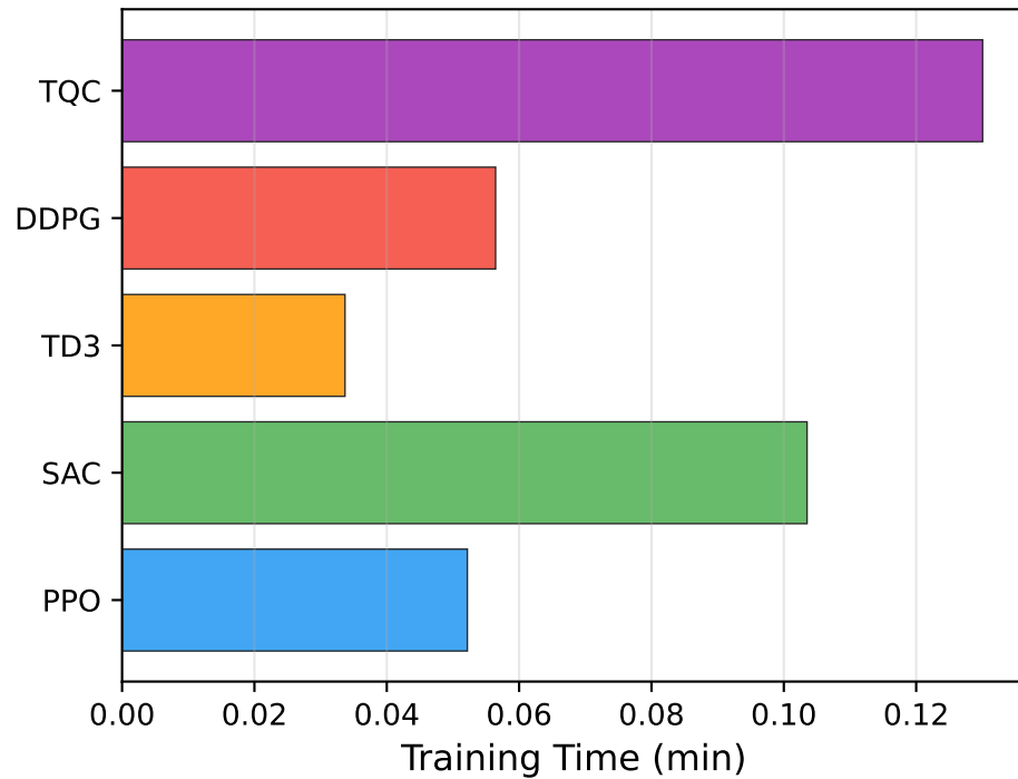
Hopper-v5
