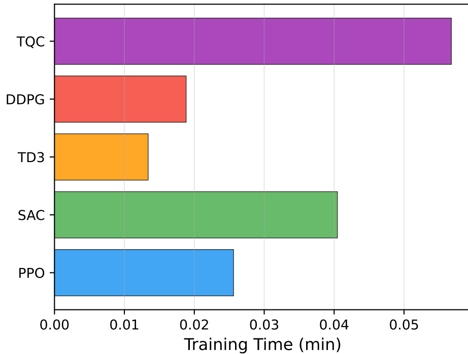
Hopper-v5
