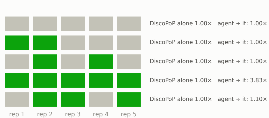
default · claude-haiku-4-5-20251001
