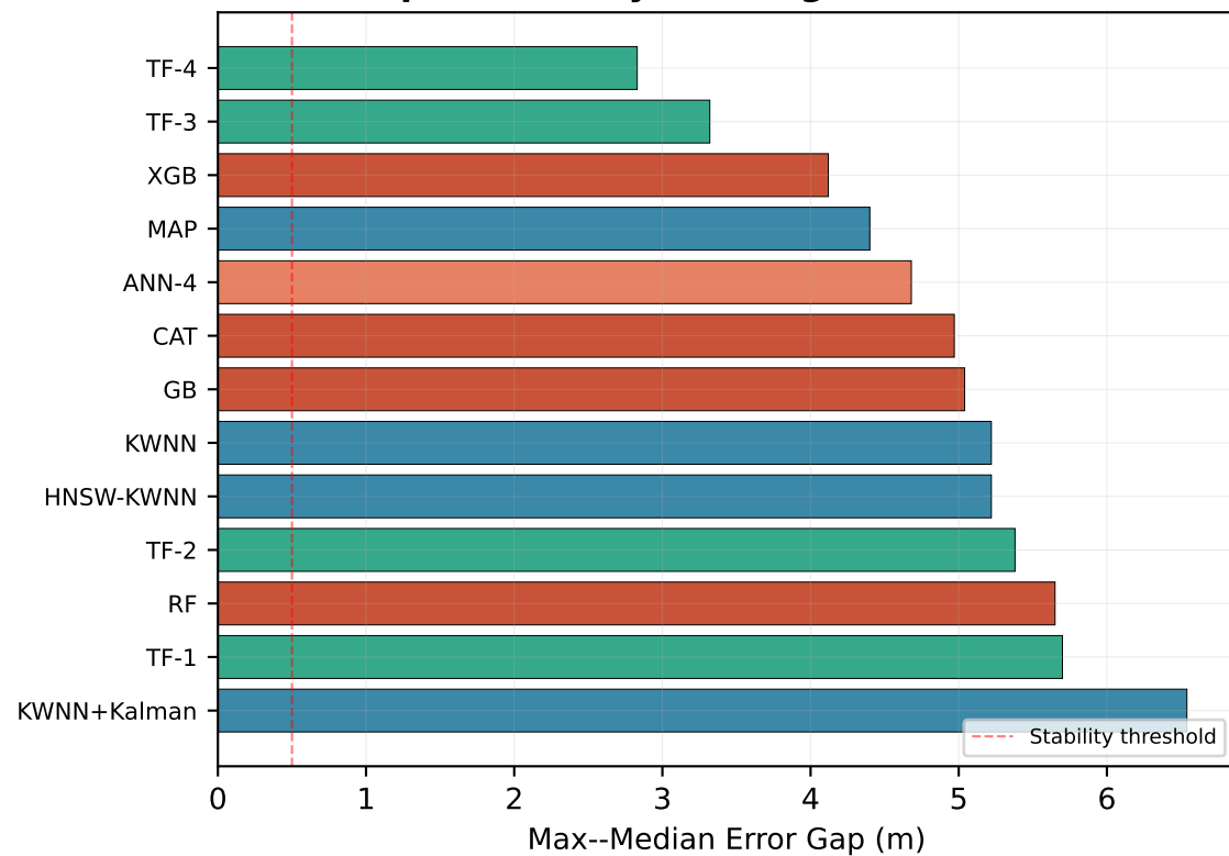
(d) Reproducibility Ranking (Lower Is Better)
