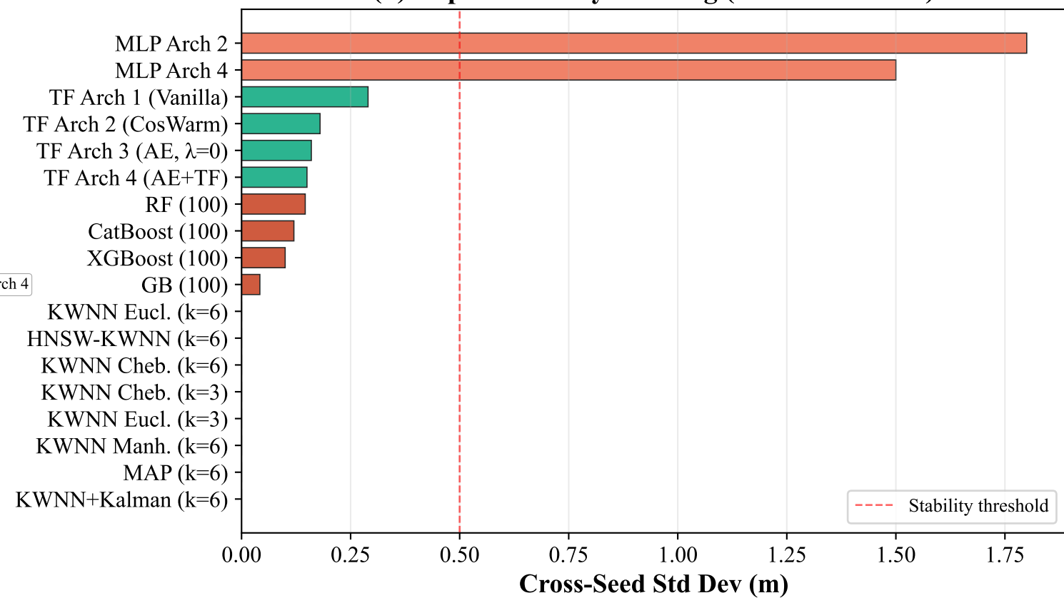
(d) Reproducibility Ranking (Lower Is Better)
