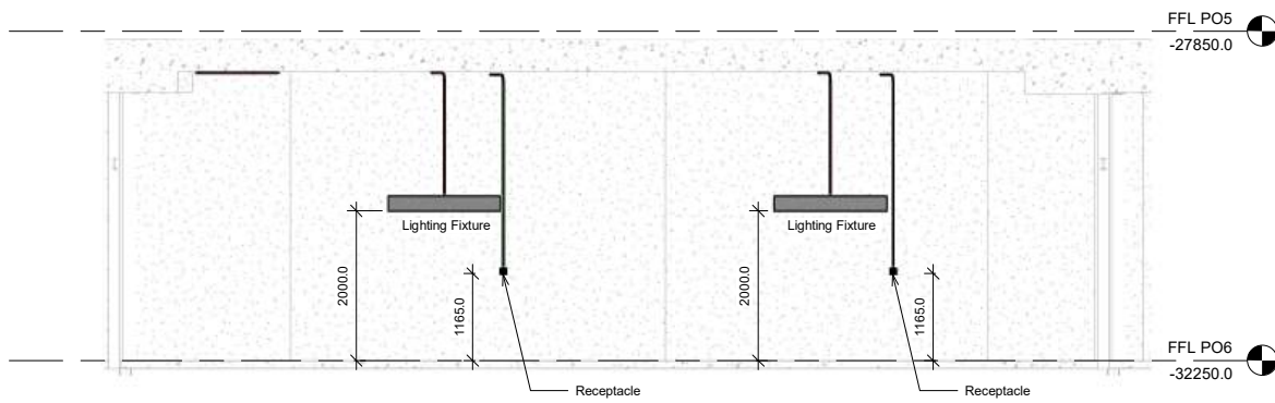
3 C/N Section 3 1 : 50
