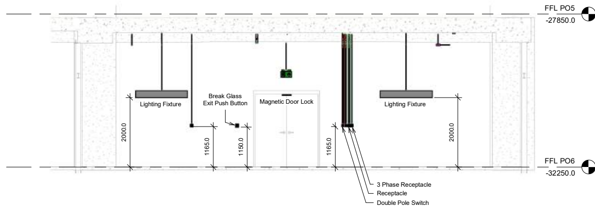
1 C/N Section 1 1 : 50
