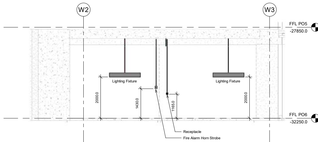
2 C/N Section 2 1 : 50
