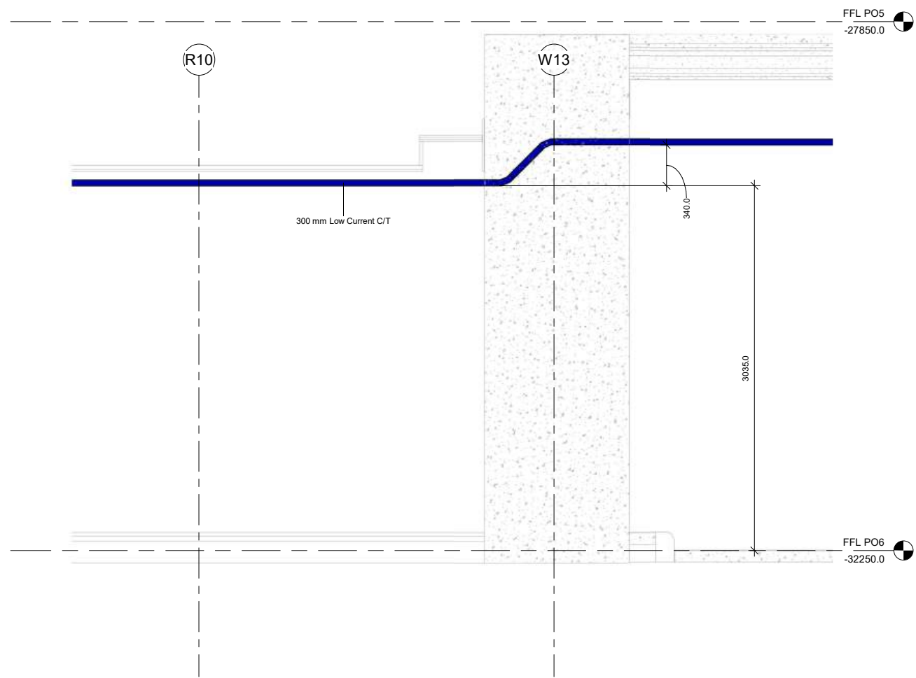
① C/T Section 1 1 : 20
