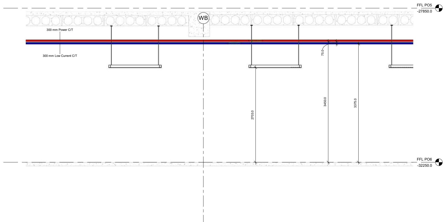
② C/T Sections 2 1 : 25
