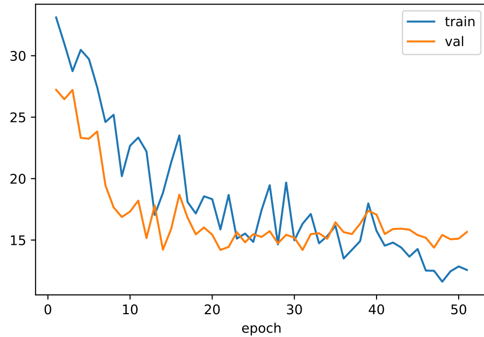
E2: Huber loss
