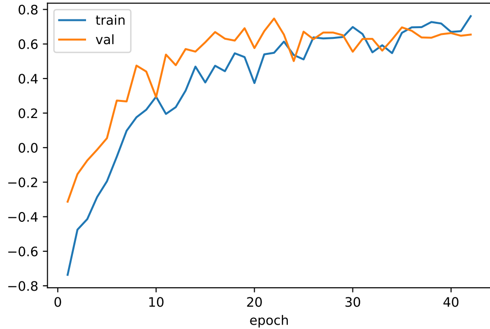
E3: R2
