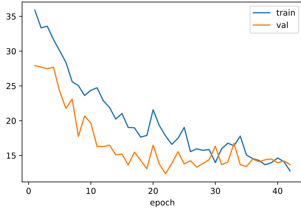
E3: MAE
