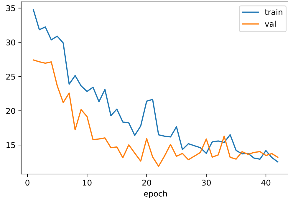
E3: Huber loss
