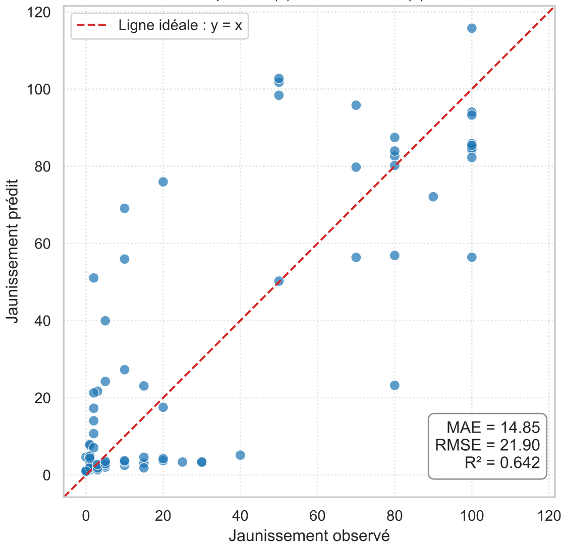
Deep Learning (E4 : SR + indices spectraux) — validation Observations vs prédictions : parcelles avec plusieurs observations 14 parcelle(s), 73 observation(s)
