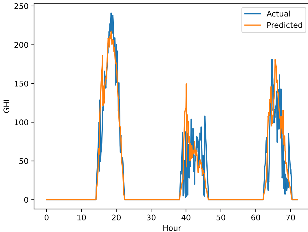
Transformer (12 Rows) GHI Pred vs Actual
