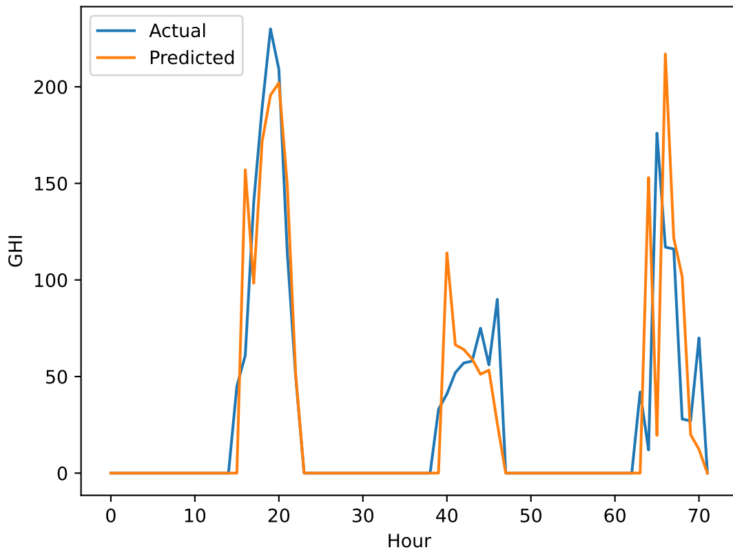
Smart Persistence GHI Pred vs Actual
