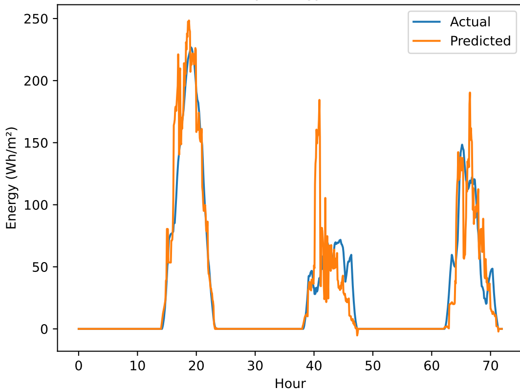
XGBoost Hourly Energy Pred vs Actual
