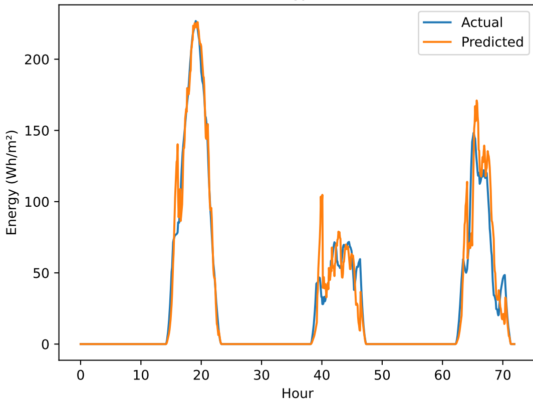
CNN+GRU Energy Pred vs Actual
