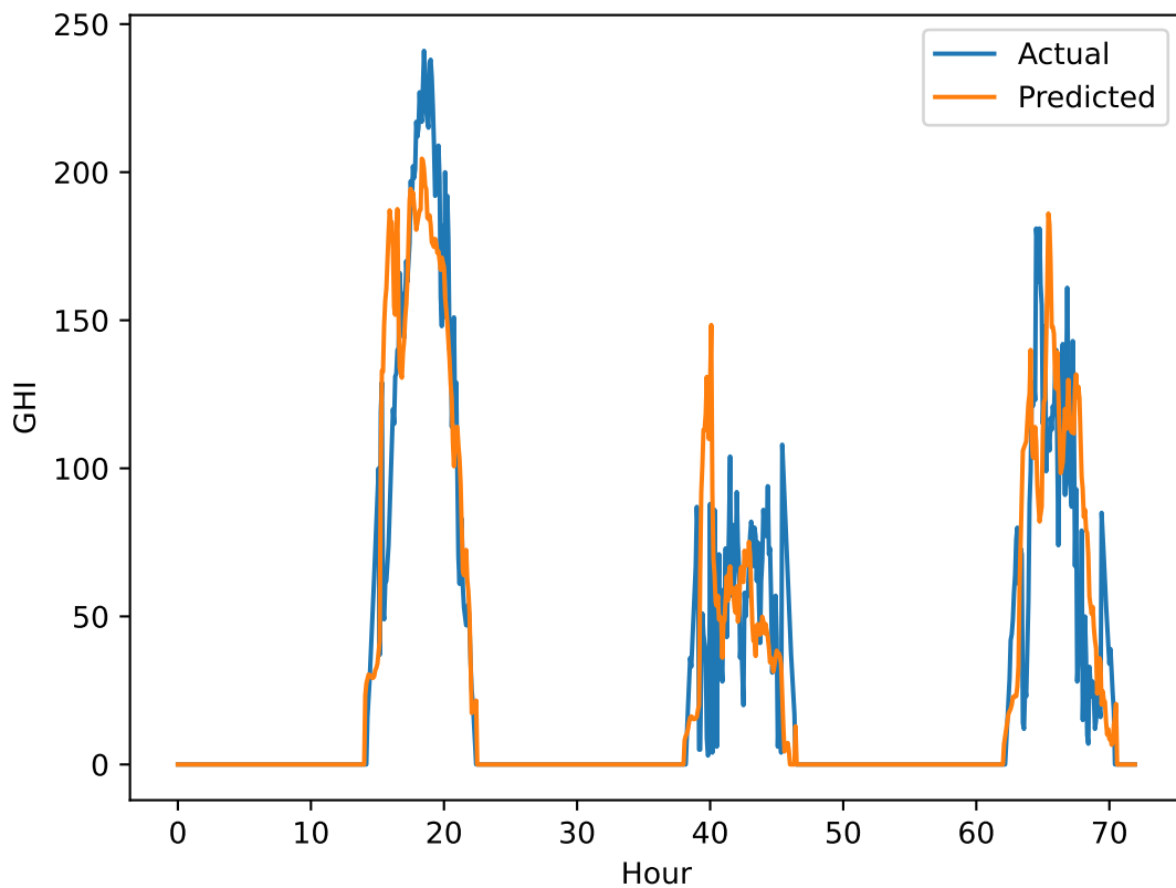
CNN+GRU GHI Pred vs Actual
