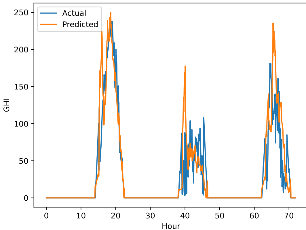
CNN+Transformer GHI Pred vs Actual
