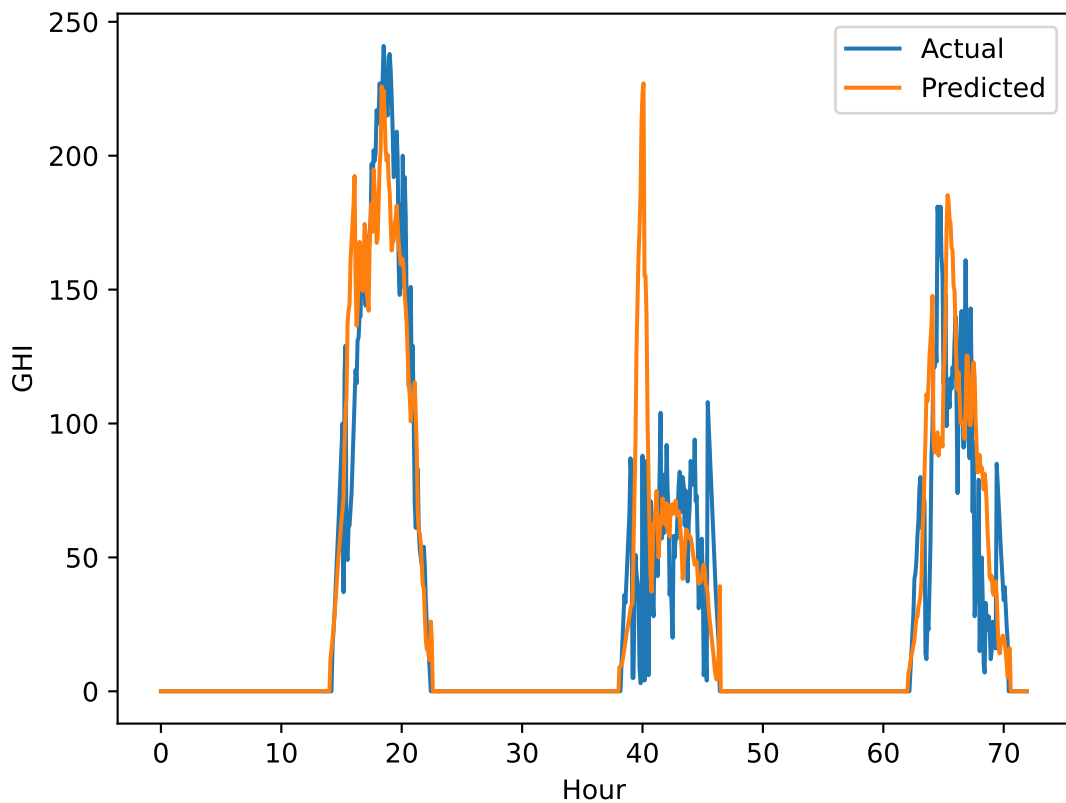
Conv3D GHI Pred vs Actual
