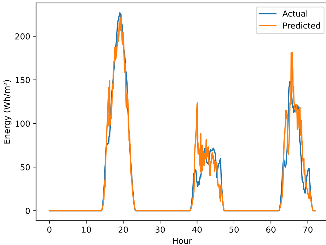
XGBoost (12 Rows) Energy Pred vs Actual
