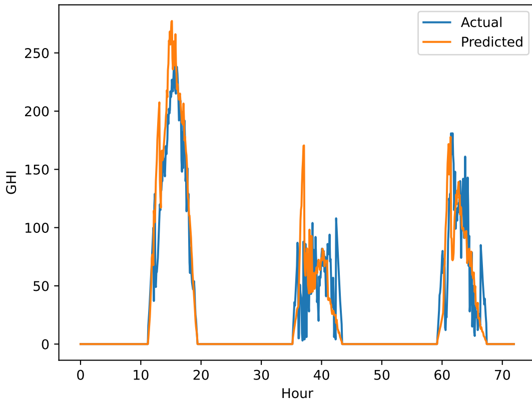
Transformer (48 Rows) GHI Pred vs Actual
