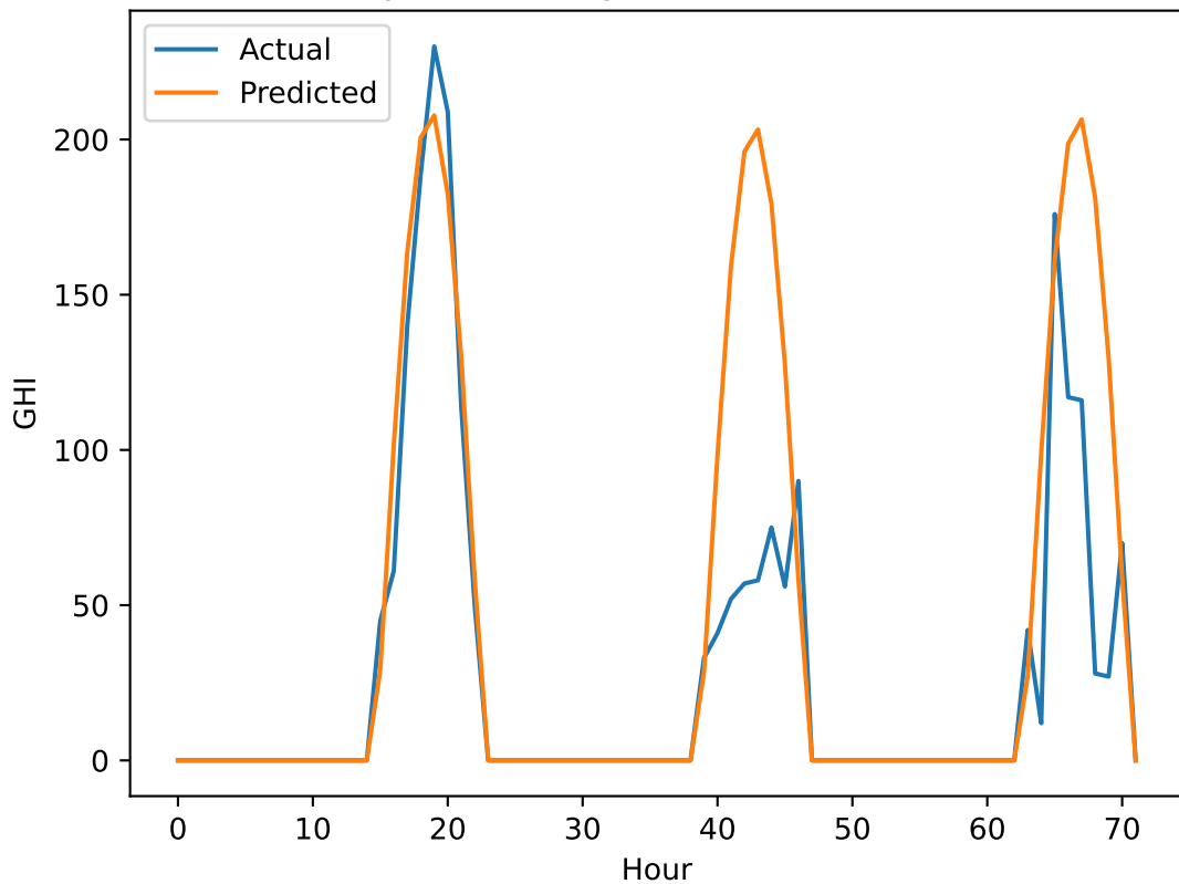
Daytime Average GHI Pred vs Actual
