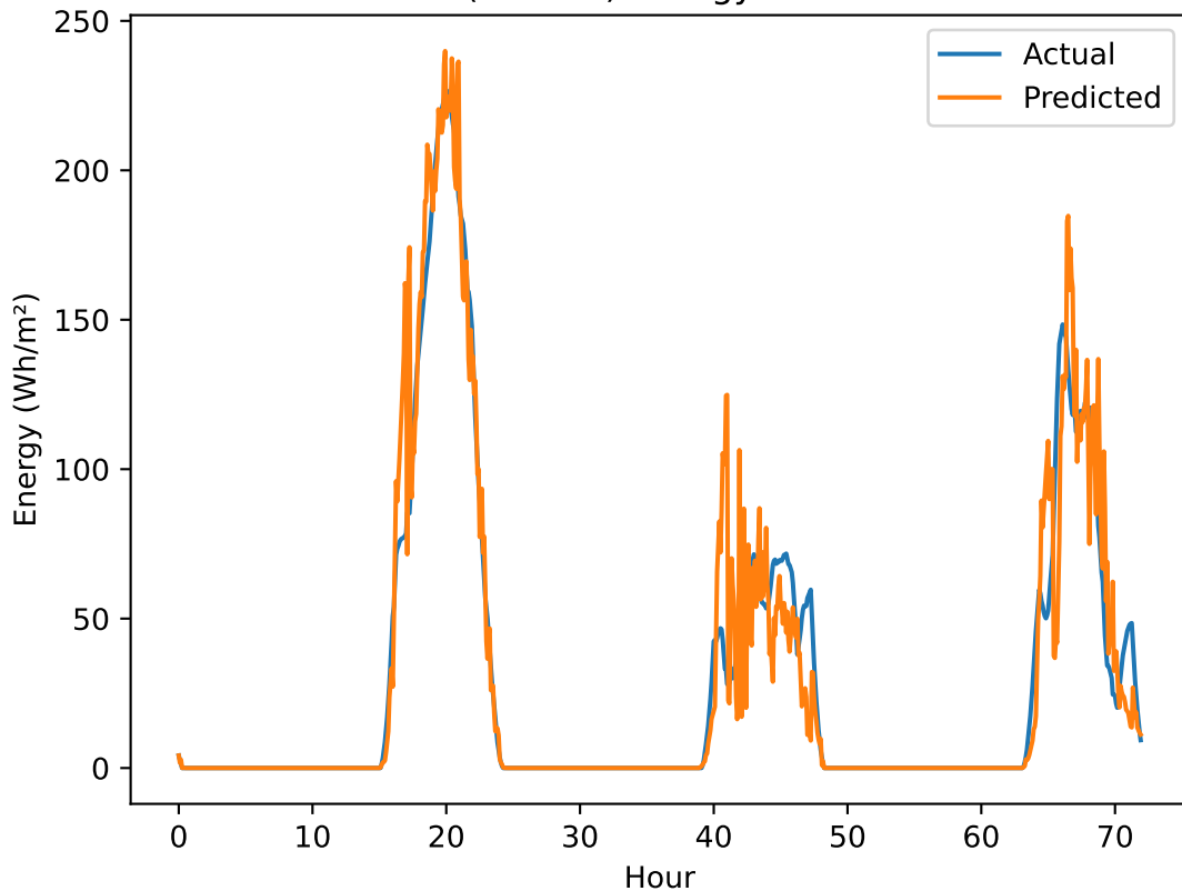
XGBoost (1 Rows) Energy Pred vs Actual
