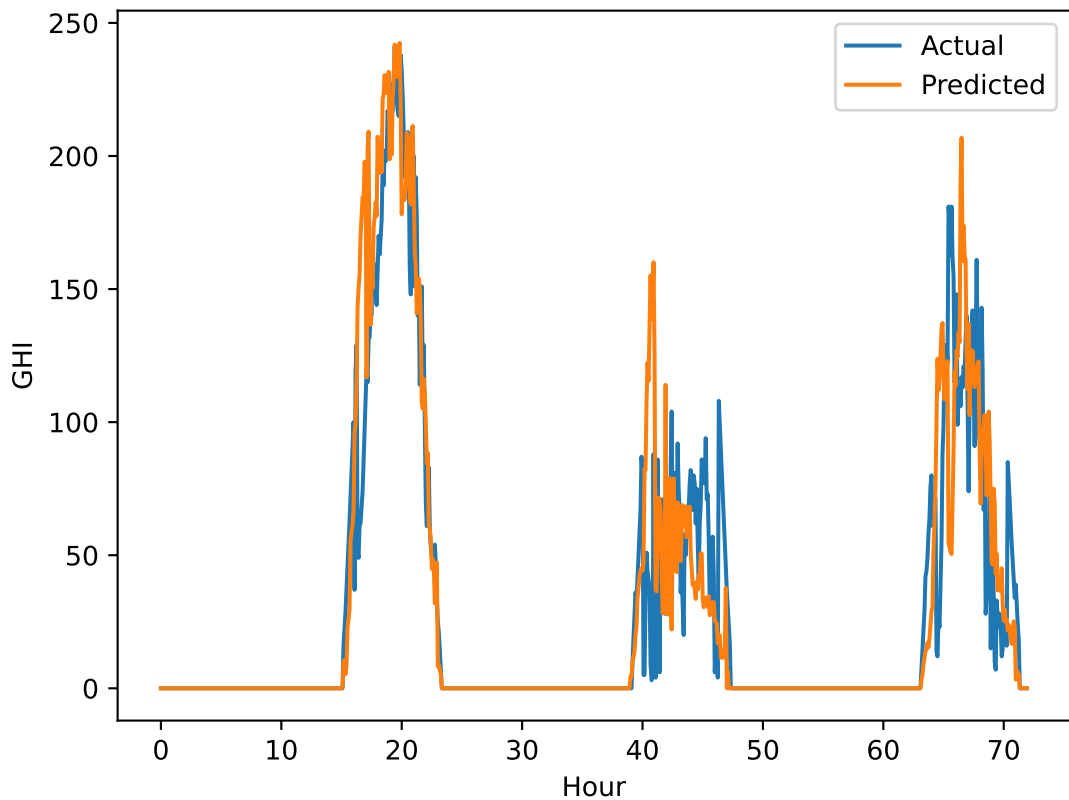
XGBoost (1 Rows) GHI Pred vs Actual
