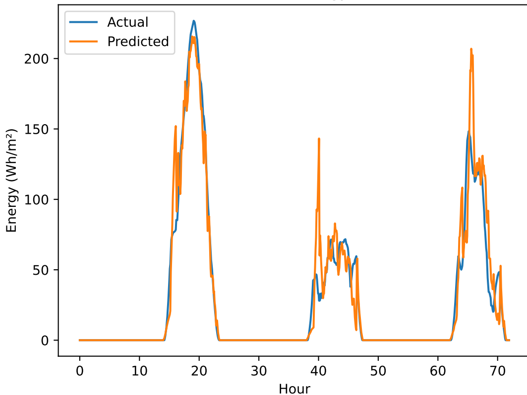
ConvLSTM (12 Rows) Energy Pred vs Actual
