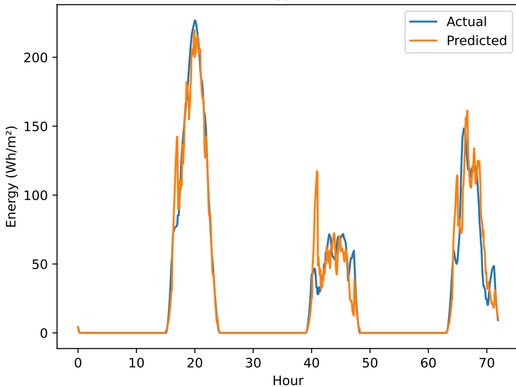
XGBoost Energy Pred vs Actual
