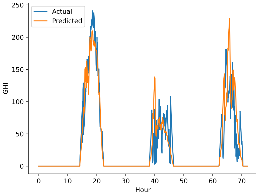
ConvGRU (12 Rows) GHI Pred vs Actual
