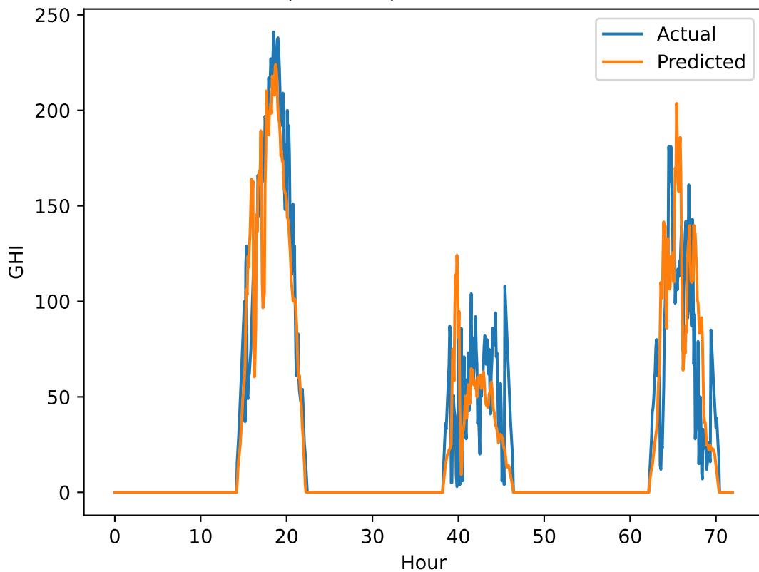
MLP (12 Rows) GHI Pred vs Actual
