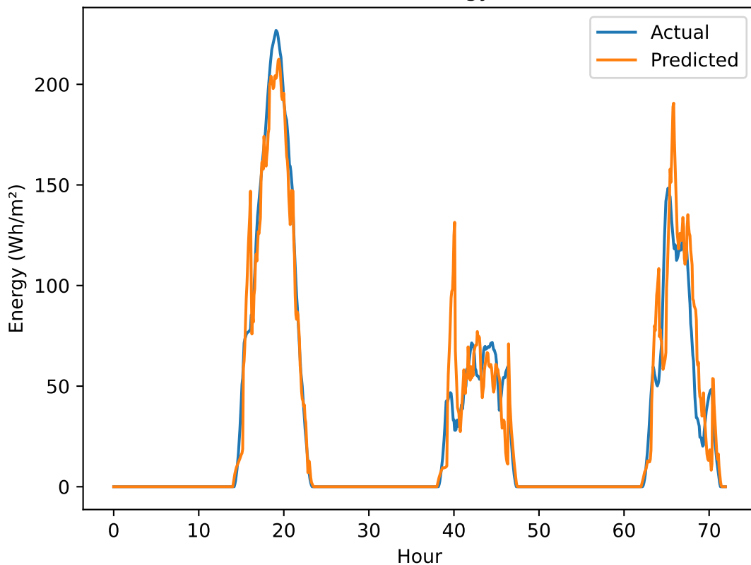
ConvGRU (12 Rows) Energy Pred vs Actual
