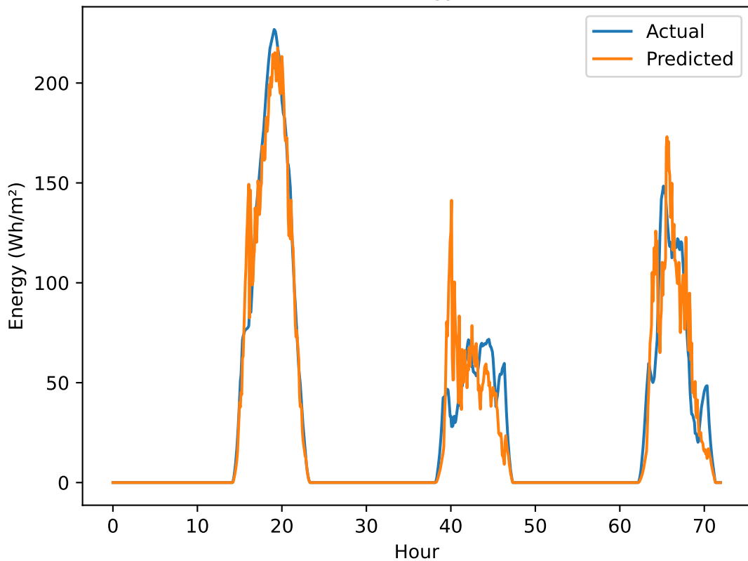
MLP (12 Rows) Energy Pred vs Actual
