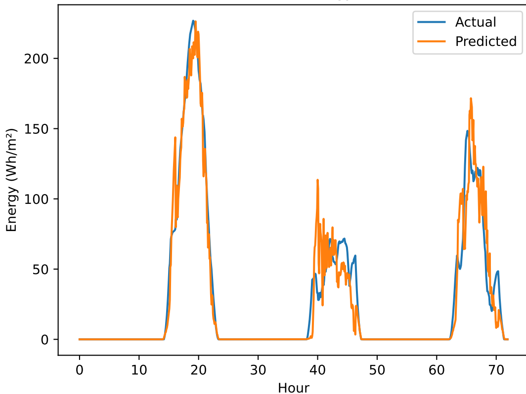
Transformer (12 Rows) Energy Pred vs Actual
