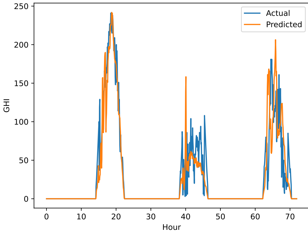
ConvGRU GHI Pred vs Actual
