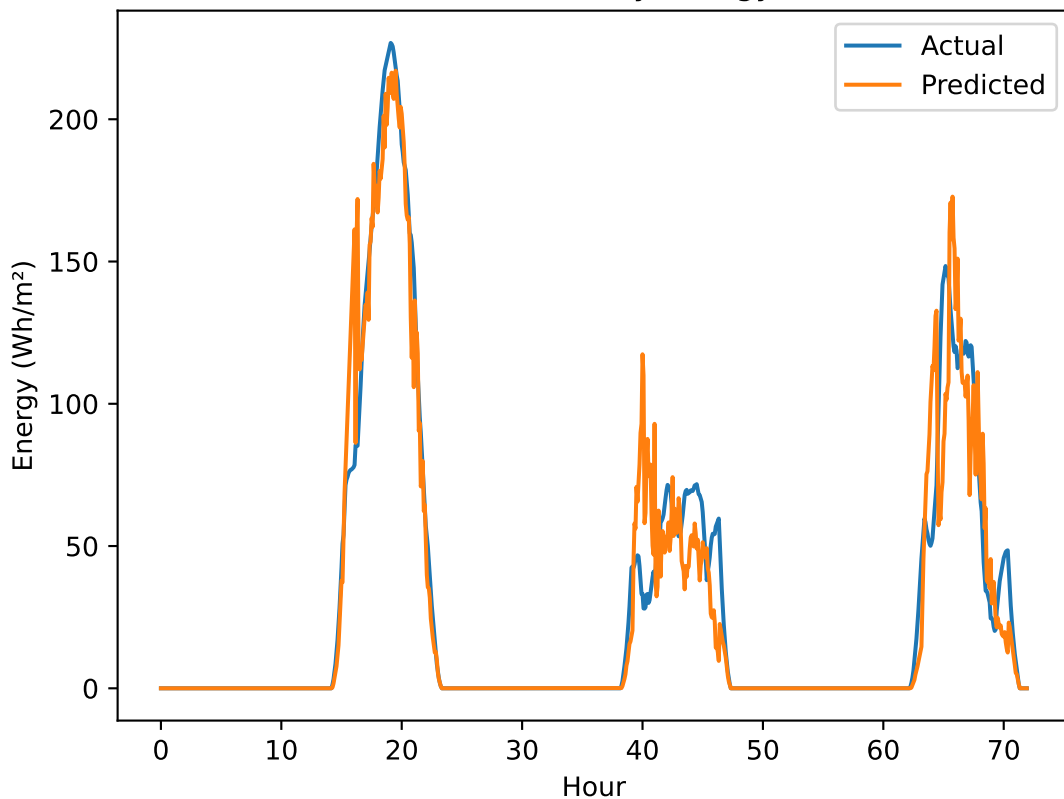
Transformer (12 Rows) Hourly Energy Pred vs Actual
