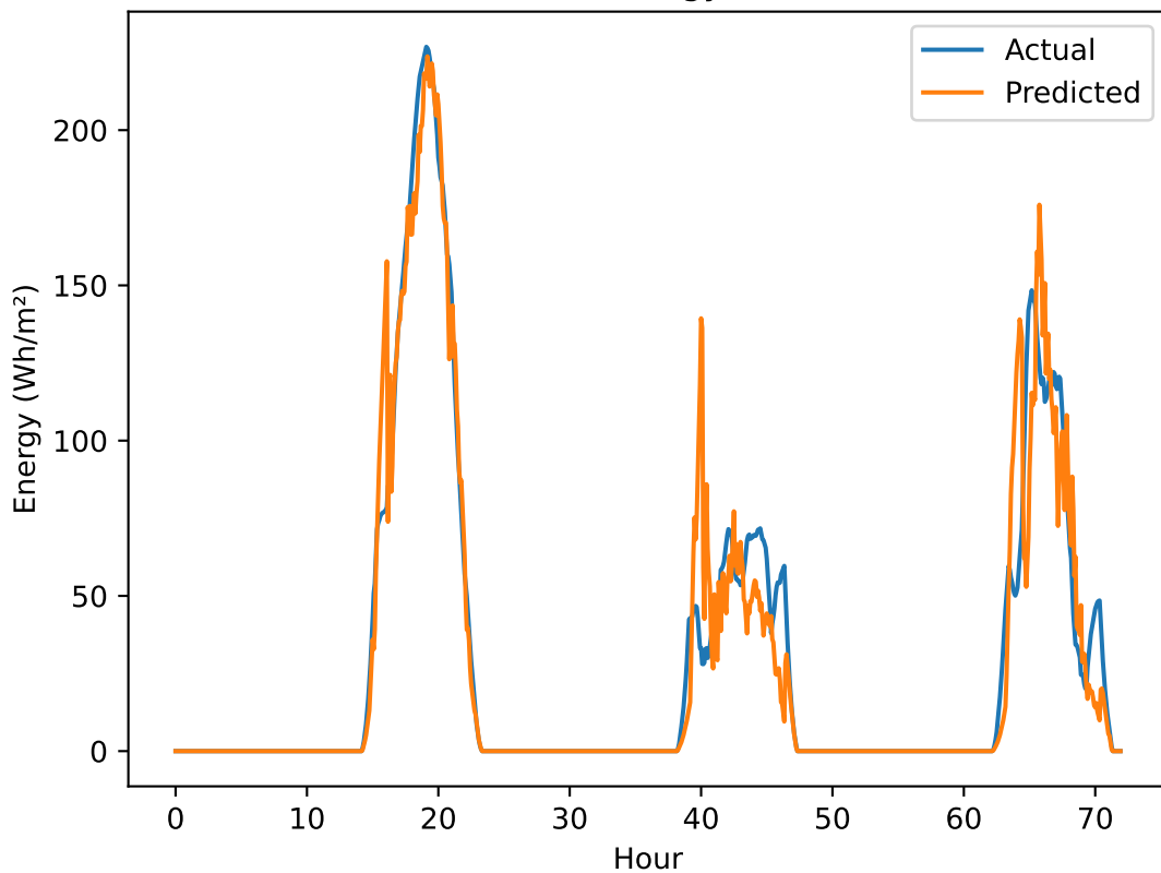
LSTM (12 Rows) Energy Pred vs Actual
