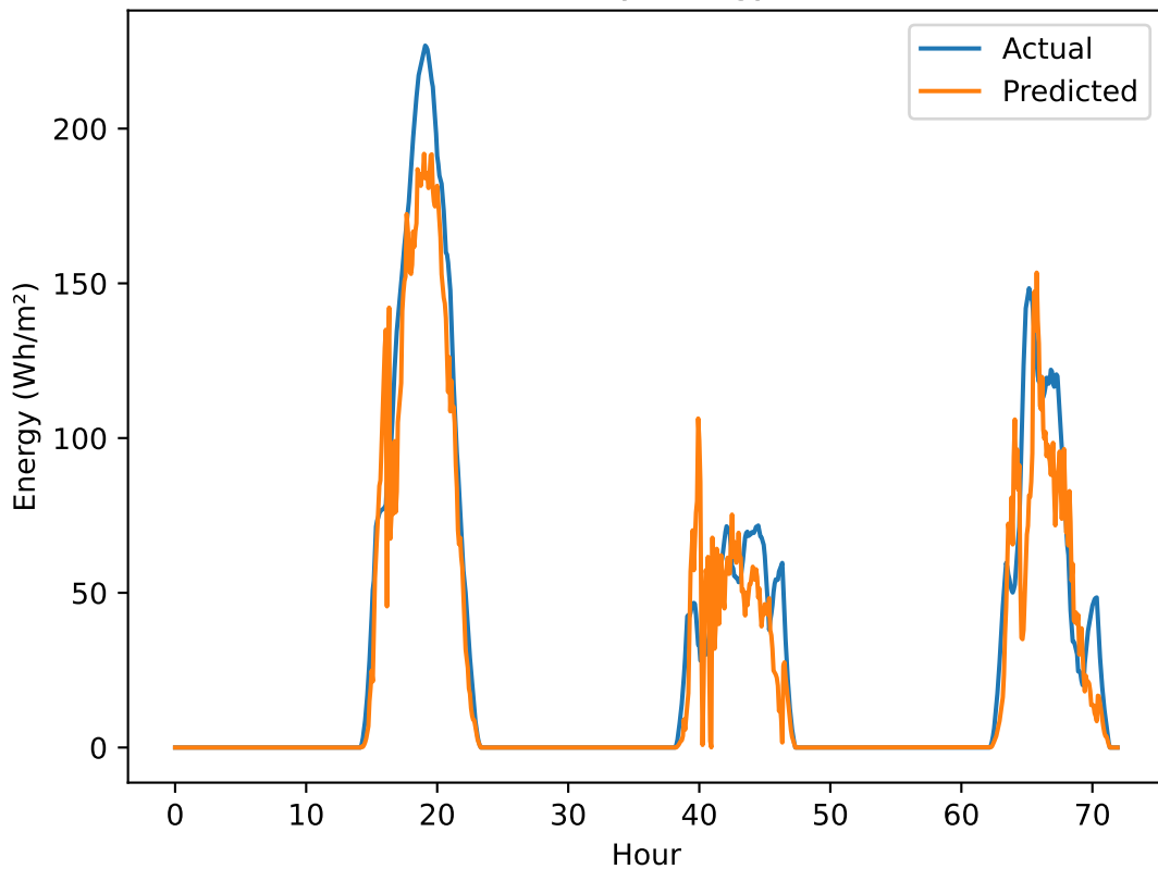
MLP (12 Rows) Hourly Energy Pred vs Actual
