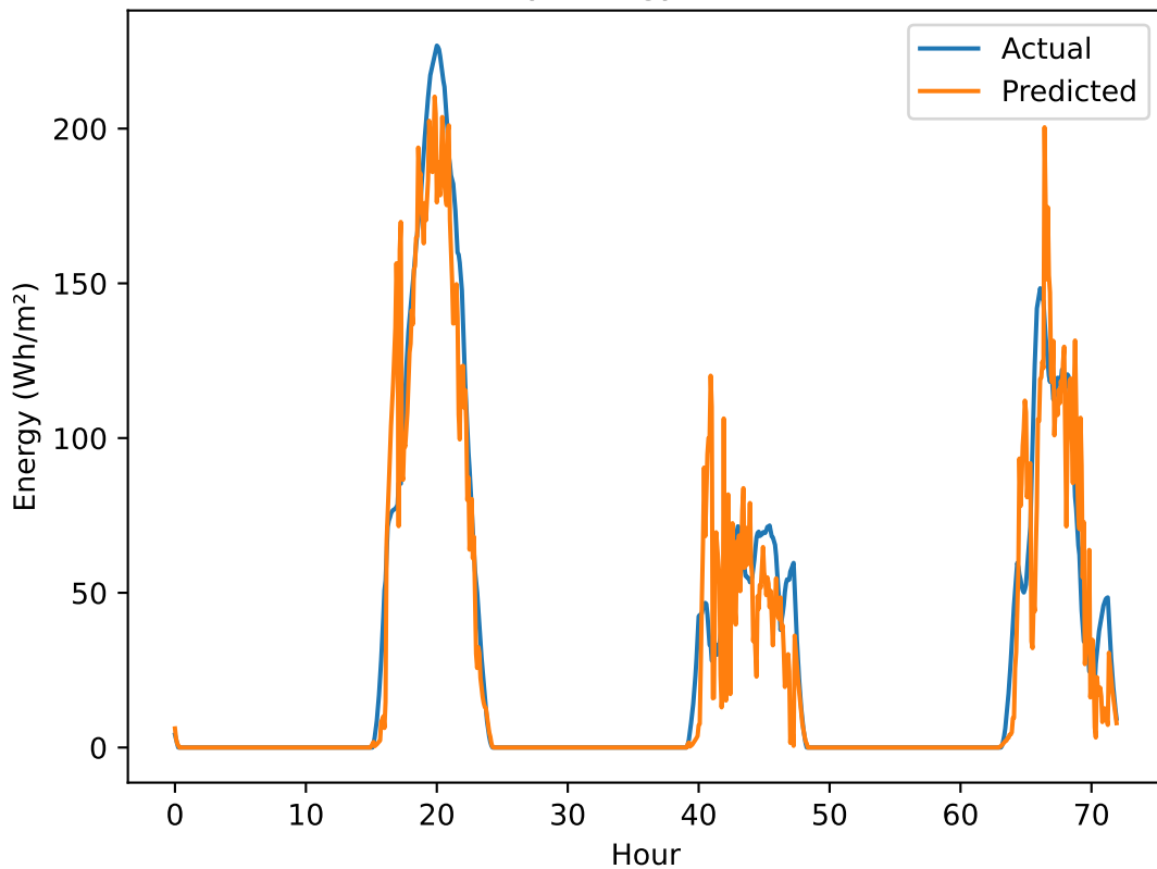
MLP Hourly Energy Pred vs Actual
