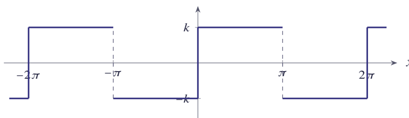
شکل ۲.۱ موج مربعی \pm k با دوره تناوب 2\pi در مثال توان
