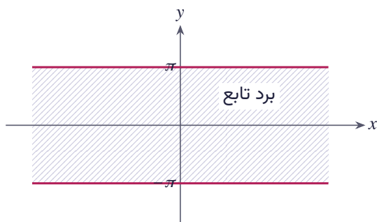
شکل ۱۰.۴ برد تابع لگاریتم: نوار -\pi < \text{Im } w \leq \pi
