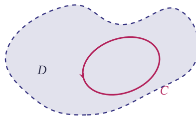
شکل ۵.۲۹ مسیر ساده بسته C در ناحیه همبند ساده D
