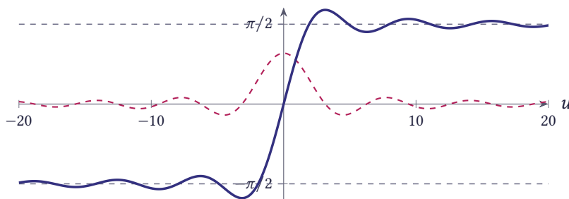
شکل ۱۰.۵۸ تابع \text{Si}(u) (خط ممتد) و تابع \sin u/u (خط چین)
