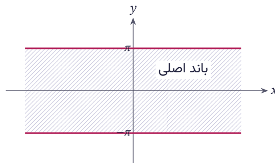
شکل ۳.۱۱ باند اصلی تابع نمایی: -\pi < y \leq \pi
