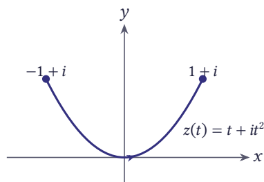
شکل ۵.۲۴ مسیر z(t) = t + it^2 ، -1 \leq t \leq 1 از -1 + i تا 1 + i
