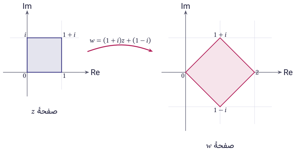
شکل ۴.۱۸ تصویر مربع واحد تحت نگاشت w = (1+i)z + (1-i)
