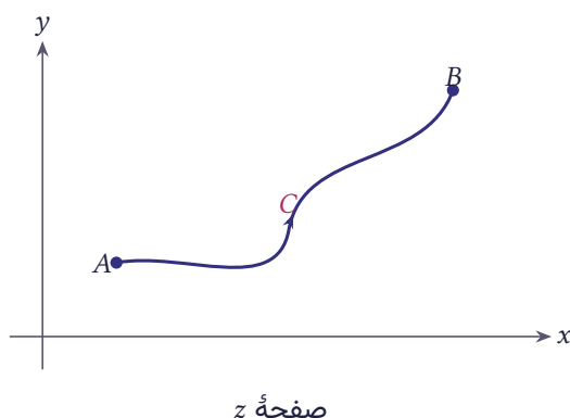
شکل ۵.۱۹ مسیر انتگرال گیری C از نقطه A تا نقطه B در صفحه z
