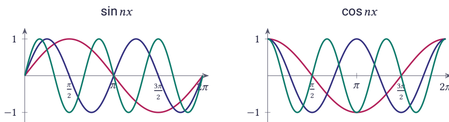
شکل ۸.۴۹ توابع \sin nx و \cos nx برای n = 1, 2, 3 در بازه [0, 2\pi]
