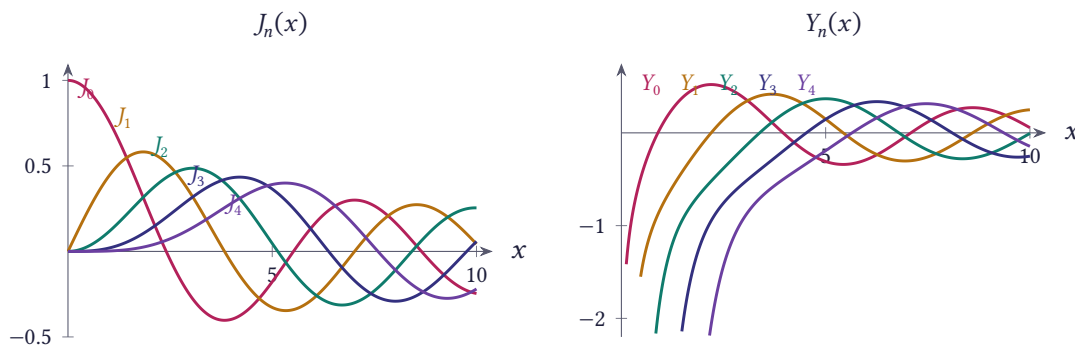
شکل ۱۳.۷۵ توابع بسل نوع اول J_0, \dots, J_4 و نوع دوم Y_0, \dots, Y_4 برای 0 < x \leq 10
