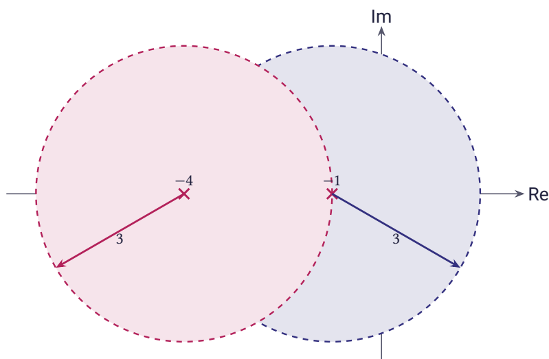
شکل ۶.۴۴ قطب‌های z = -4 و z = -1 تابع f(z) = \frac{z}{(z+1)(z+4)^3}
