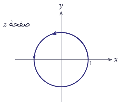
شکل ۵.۲۲ مسیر z(t) = e^{it} , 0 \leq t \leq 2\pi (دایره واحد)
