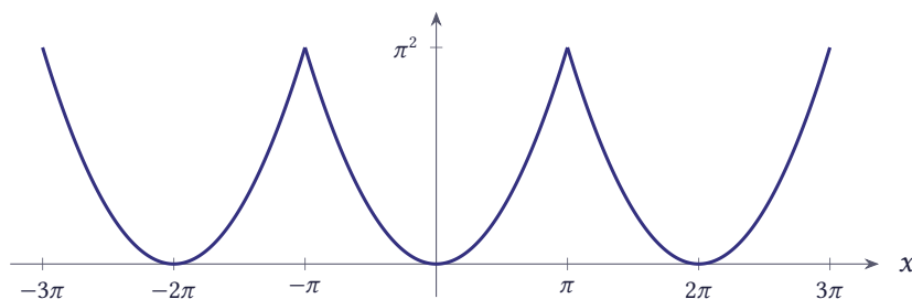
شکل ۸.۵۳ تابع f(x) = x^2 روی [-\pi, \pi] با ادامه متناوب
