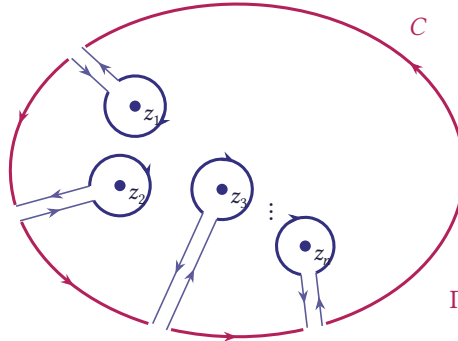
شکل ۵.۳۷ مسیر \Gamma برای اثبات: C ، دایره‌های C_1, \dots, C_n و پیوندها
