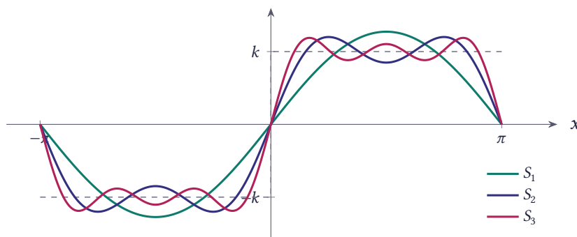
شکل ۸.۵۱ مجموع‌های جزئی S_1 ، S_2 و S_3 سری فوریه موج مربعی (خط چین خود موج مربعی است)
