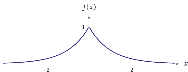
شکل ۱۰.۶۰ تابع f(x) = e^{-|x|}
