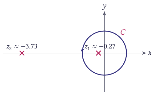
شکل ۷.۴۷ دایره واحد و قطب‌های z_1 \approx -0.27 (داخل) و z_2 \approx -3.73 (بیرون)
