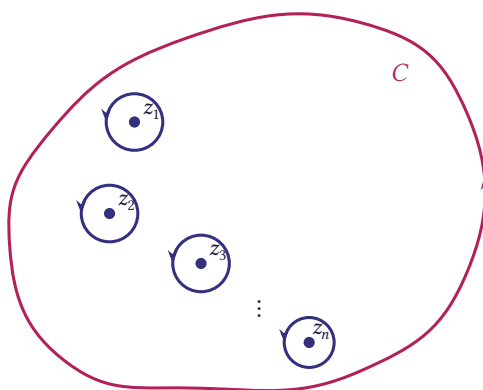
شکل ۶.۴۰ مسیر C و نقاط تکین z_1, \dots, z_n در داخل آن؛ حول هر نقطه دایره‌ای کوچک رسم شده است
