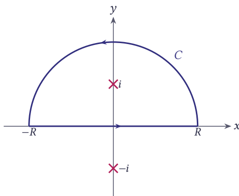
شکل ۵.۳۳ مسیر نیم‌دایره در نیم‌صفحه بالایی؛ قطب‌ها در z = \pm i
