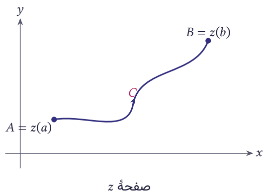
شکل ۵.۲۰ مسیر C با جهت از A = z(a) به B = z(b)
