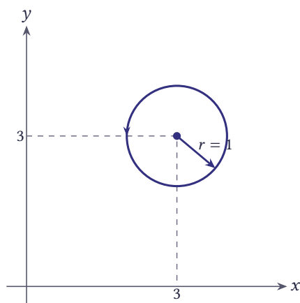
شکل ۵.۳۹ مسیر تمرین ۴: دایره‌ای به مرکز 3 + 3i و شعاع r = 1
