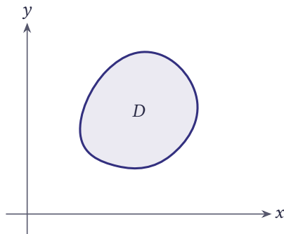
شکل ۲.۸ میدان D در صفحه مختلط
