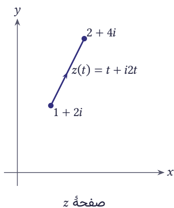
شکل ۵.۲۱ مسیر z(t) = t + i2t , 1 \leq t \leq 2
