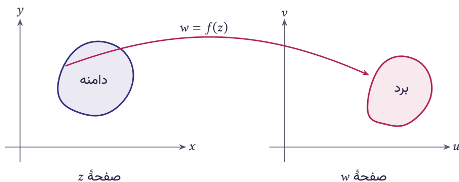
شکل ۲.۵ تابع مختلط w = f(z) نقاط دامنه در صفحه z را به نقاط برد در صفحه w می‌نگارد
