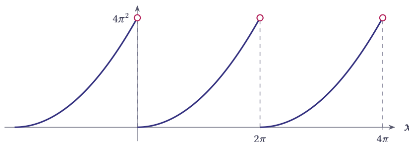
شکل ۸.۵۴ تابع f(x) = x^2 روی [0, 2\pi] با ادامه متناوب
