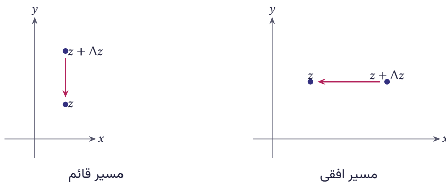
شکل ۲.۱۰ دو مسیر نزدیک شدن به z : راستای قائم ( \Delta z = i\Delta y ) و راستای افقی ( \Delta z = \Delta x )
