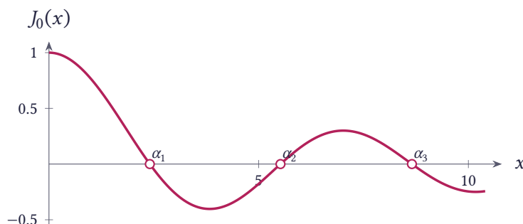
شکل ۱۳.۷۶ تابع J_0(x) و ریشه‌های آن \alpha_1, \alpha_2, \alpha_3
