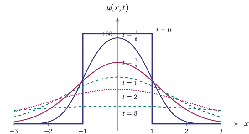
شکل ۱۲.۷۰ توزیع دما u(x, t) در لحظه‌های t = 0, \frac{1}{8}, \frac{1}{2}, 1, 2 و ۸ برای پالس اولیه U_0 = 100 و c = 1
