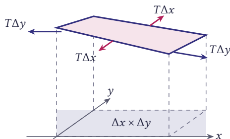
شکل ۱۳.۷۱ المان \Delta x \times \Delta y از غشاء مرتعش و نیروهای کششی T\Delta x و T\Delta y وارد بر آن
