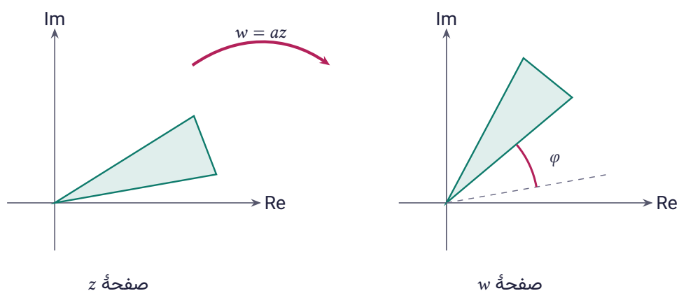
شکل ۴.۱۶ دوران w = az با |a| = 1 : ناحیه‌ای از صفحه z به اندازه \varphi = \arg a حول مبدأ می‌چرخد
