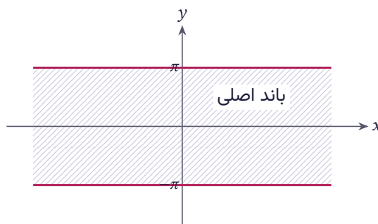
شکل ۳.۱۳ باند اصلی توابع هذلولی‌گون: -\pi < y \leq \pi
