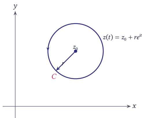
شکل ۵.۳۱ دایره C به مرکز z_0 و شعاع r
