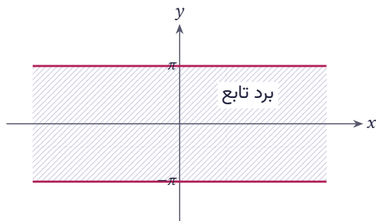
شکل ۳.۱۴ برد تابع لگاریتم: نوار -\pi < \operatorname{Im} w \leq \pi
