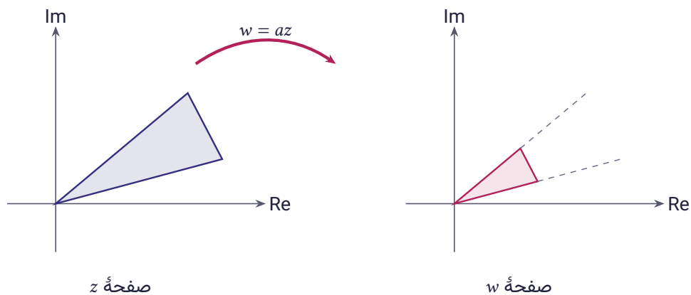
شکل ۴.۱۷ انقباض w = az با 0 < a < 1 ؛ برای a > 1 نگاشت یک انبساط است
