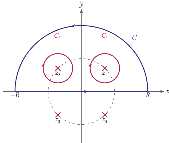
شکل ۵.۳۵ مسیر نیم‌دایره و دایره‌های C_1 و C_2 حول قطب‌های z_1 و z_2 ؛ قطب‌های z_3 و z_4 در نیم‌صفحه پایینی
