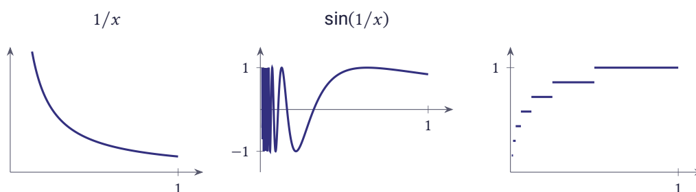
شکل ۸.۵۵ توابعی که شرایط دریشه را ندارند: 1/x (نامحدود)، \sin(1/x) (بی‌نهایت ماکزیمم و مینیمم) و تابع پله‌ای با بی‌نهایت پله
