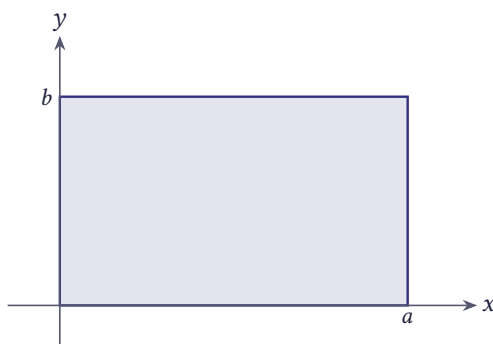
شکل ۱۳.۷۲ ناحیه مستطیلی 0 \leq x \leq a, 0 \leq y \leq b
