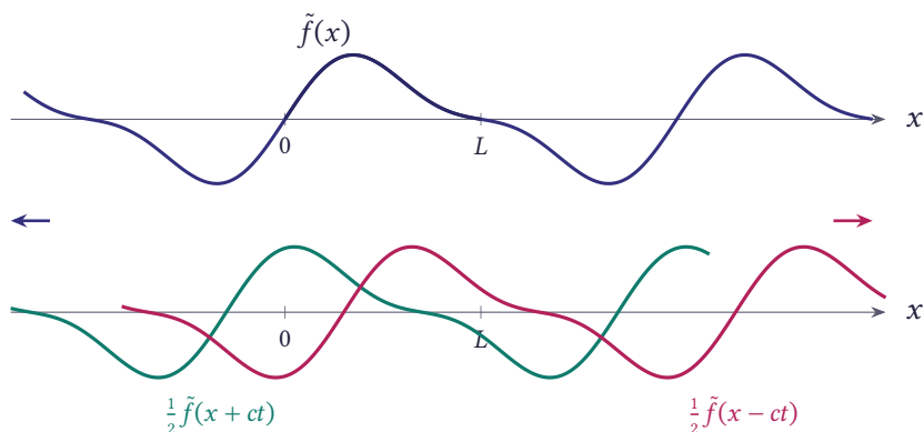
شکل ۱۱.۶۶ ادامه فرد و متناوب \tilde{f}(x) و دو موج \frac{1}{2}\tilde{f}(x+ct) و \frac{1}{2}\tilde{f}(x-ct) که در دو جهت مخالف حرکت می‌کنند
