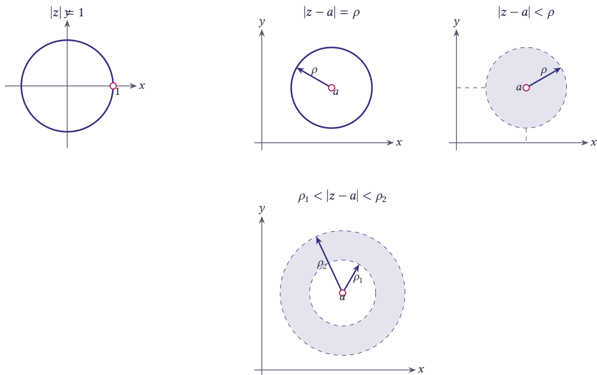
شکل ۲.۶ مکان‌های هندسی مهم: دایره، \rho -همسایگی نقطه a و ناحیه حلقوی
