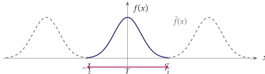
شکل ۱۰.۵۷ تابع غیرتناوبی f(x) و ادامه تناوب آن \tilde{f}(x) با دوره تناوب T
