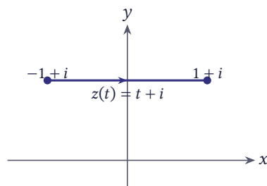
شکل ۵.۲۵ مسیر z(t) = t + i ، -1 \leq t \leq 1 از -1 + i تا 1 + i
