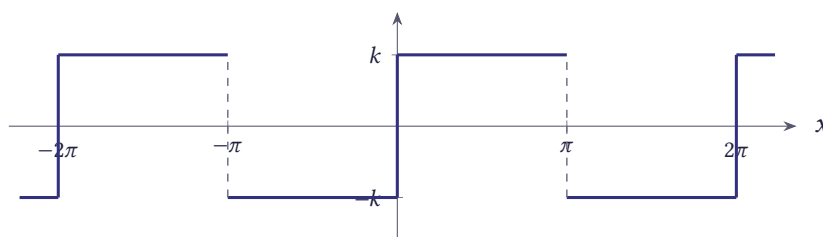
شکل ۹.۵۶ موج مربعی \pm k با دوره تناوب 2\pi در مثال توان
