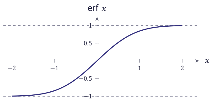
شکل ۱۲.۶۹ نمودار تابع خطا \operatorname{erf}(x) برای -2 \leq x \leq 2
