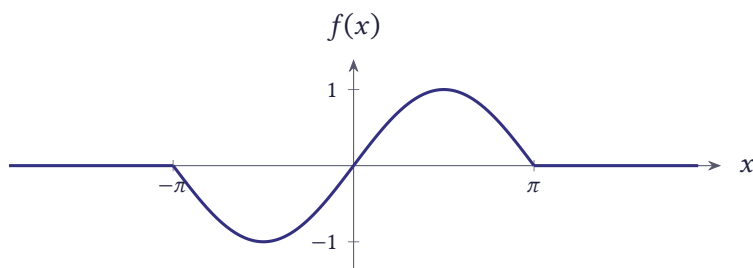
شکل ۱۰.۶۱ تابع f(x) = \sin x برای |x| \leq \pi و صفر در بیرون
