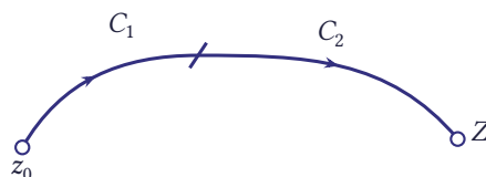
شکل ۵.۲۶ مسیر C از z_0 تا Z که به دو تکه C_1 و C_2 تقسیم شده است
