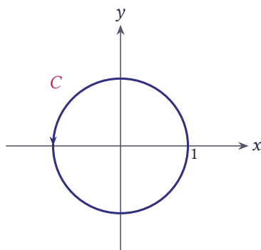
شکل ۷.۴۶ دایره واحد z = e^{it} , 0 \leq t \leq 2\pi
