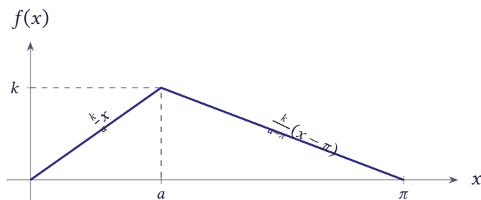
شکل ۱۱.۶۴ توزیع اولیه مثلثی f(x) با قله k در x = a
