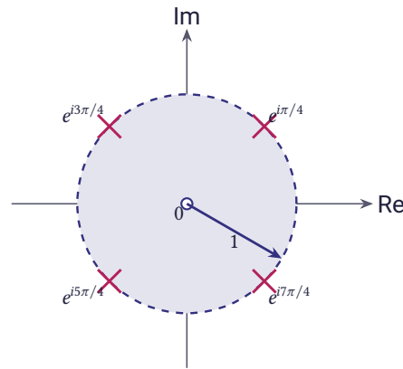
شکل ۶.۴۱ چهار قطب z^4 + 1 = 0 روی دایره واحد؛ شعاع همگرایی سری حول مبدأ برابر ۱ است
