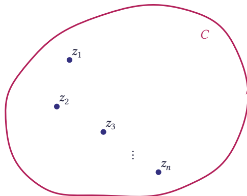
شکل ۵.۳۶ مسیر C و نقاط غیرتحلیلی z_1, \dots, z_n در داخل آن
