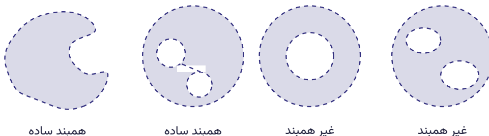
شکل ۵.۲۸ ناحیه‌های همبند ساده و غیر همبند
