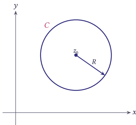
شکل ۵.۳۸ دایره C به مرکز z_0 و شعاع R
