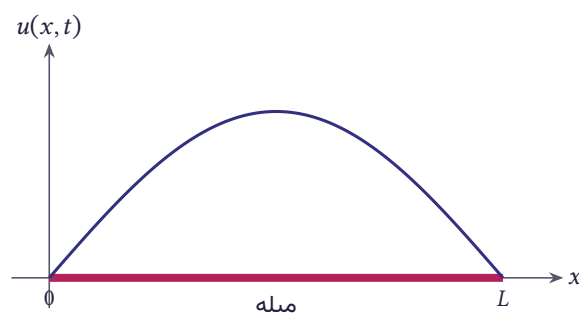
شکل ۱۲.۶۸ میله یک بعدی 0 \leq x \leq L با توزیع دمای u(x, t)
