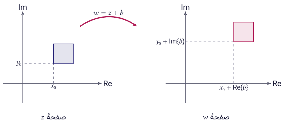
شکل ۴.۱۵ انتقال w = z + b : ناحیه‌ای از صفحه z بدون تغییر شکل به اندازه b جابه‌جا می‌شود
