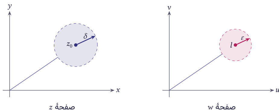
شکل ۲.۷ تعریف حد: دایره \delta -همسایگی z_0 در صفحه z و دایره \epsilon -همسایگی l در صفحه w
