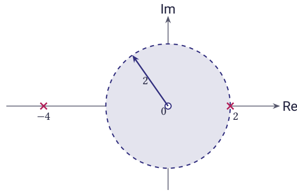
شکل ۶.۴۲ قطب‌های z = 2 و z = -4 ؛ دایره همگرایی حول مبدأ شعاع ۲ دارد
