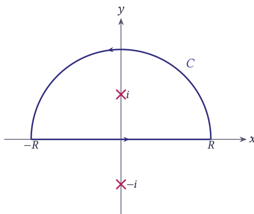
شکل ۷.۴۵ مسیر نیم‌دایره بالایی؛ قطب مرتبه دوم z = i داخل مسیر و z = -i بیرون آن است
