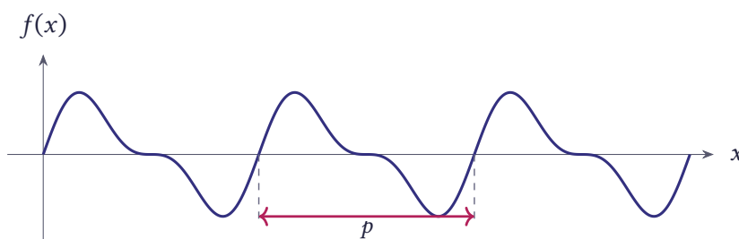
شکل ۸.۴۸ تابعی متناوب با دوره تناوب p
