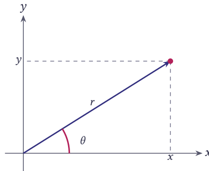
شکل ۱۳.۷۳ مختصات قطبی: x = r \cos \theta , y = r \sin \theta
