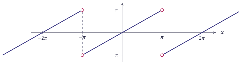
شکل ۸.۵۲ موج دندانه‌اره‌ای f(x) = x روی [-\pi, \pi] با ادامه متناوب
