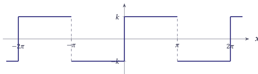
شکل ۸.۵۰ موج مربعی f(x) با دوره تناوب 2\pi و مقادیر \pm k
