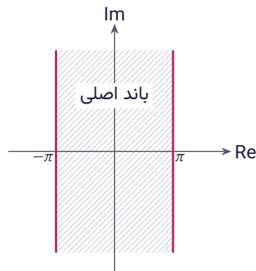
شکل ۳.۱۲ باند اصلی توابع \cos z و \sin z : -\pi < x \leq \pi
