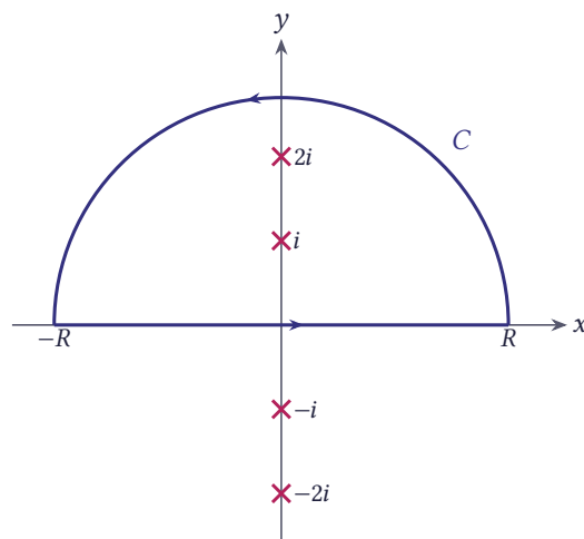
شکل ۵.۳۴ مسیر نیم‌دایره؛ قطب‌ها در z = \pm 2i و z = \pm i
