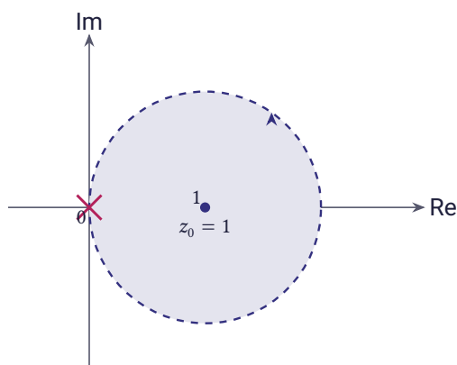
شکل ۶.۴۳ ناحیه همگرایی سری حول z_0 = 1 دایره‌ای به شعاع ۱ است (تا قطب z = 0 )
