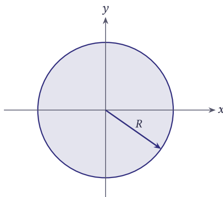
شکل ۱۳.۷۴ غشاء دایره‌ای به شعاع R
