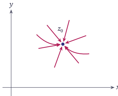
شکل ۲.۹ نزدیک شدن به نقطه z_0 از تمام جهات
