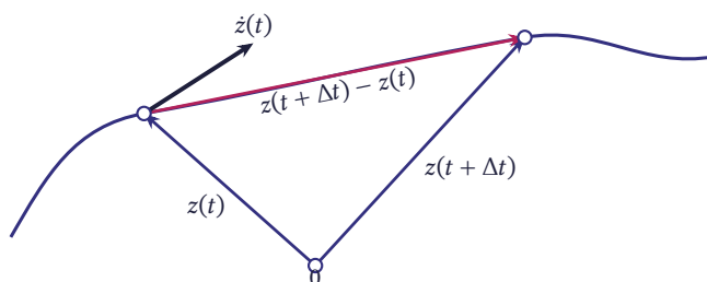
شکل ۵.۲۳ مشتق مسیر \dot{z}(t) به عنوان حد \frac{z(t+\Delta t)-z(t)}{\Delta t}
