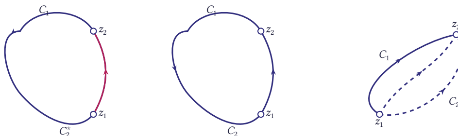
شکل ۵.۳۰ مسیرهای C_1 ، C_2 و C_2^* (مسیر C_2 با جهت معکوس) میان z_1 و z_2
