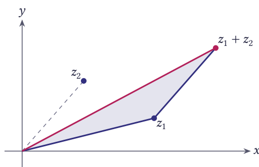
شکل ۱.۳ نامساوی مثلثی: مثلثی با رئوس 0 ، z_1 و z_1 + z_2
