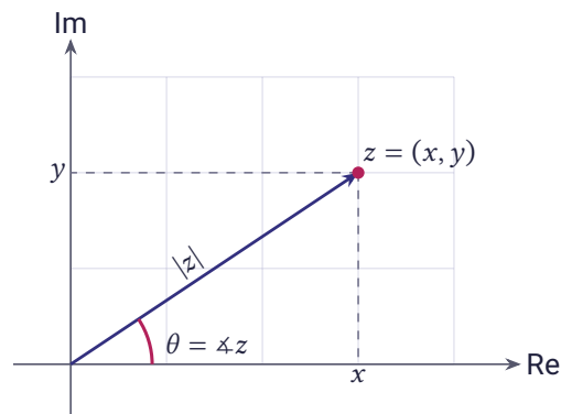
شکل ۱.۱ نمایش عدد مختلط z = (x, y) در صفحه مختلط؛ اندازه |z| و آرگومان \theta
