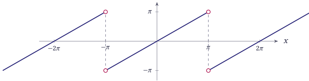
شکل ۸.۵ موج دندانه‌اره‌ای f(x) = x روی [-\pi, \pi] با ادامه متناوب
