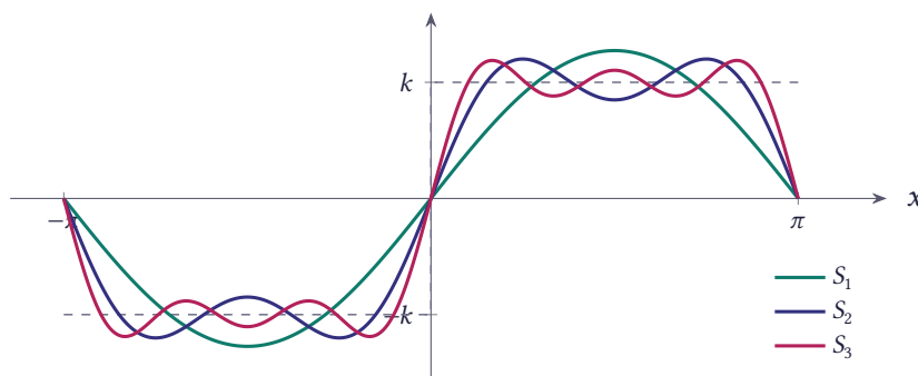
شکل ۸.۴ مجموع‌های جزئی S_1 ، S_2 و S_3 سری فوریه موج مربعی (خط چین خود موج مربعی است)
