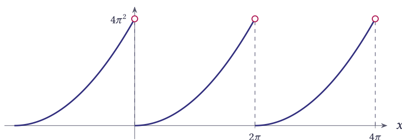
شکل ۸.۷ تابع f(x) = x^2 روی [0, 2\pi] با ادامهٔ متناوب
