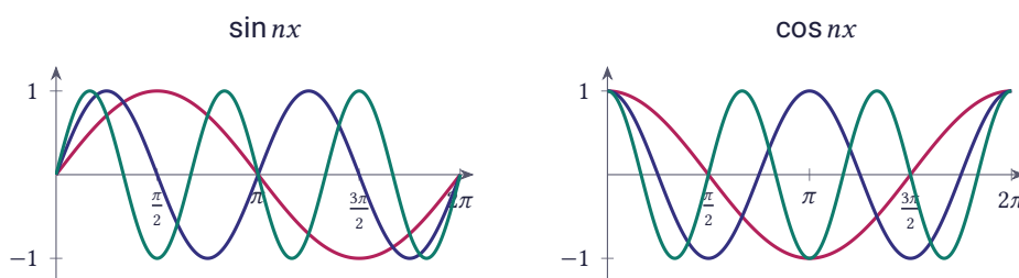
شکل ۸.۲ توابع \sin nx و \cos nx برای n = 1, 2, 3 در بازه [0, 2\pi]
