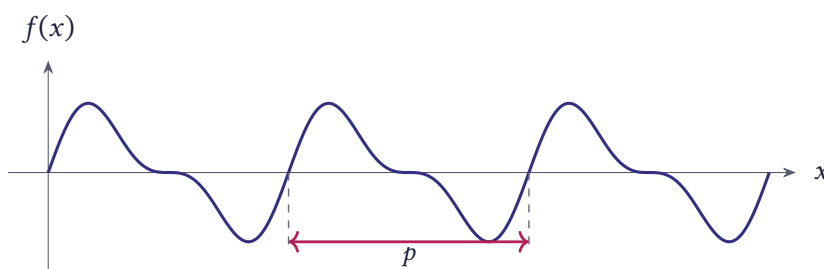
شکل ۸.۱ تابعی متناوب با دوره تناوب p
