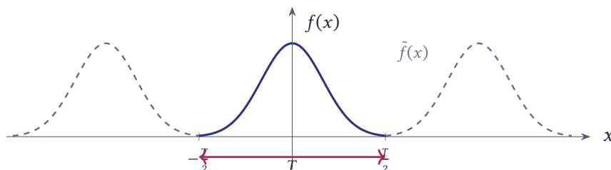
شکل ۱۰.۱ تابع غیرتناوبی f(x) و ادامه متناوب آن \tilde{f}(x) با دوره تناوب T
