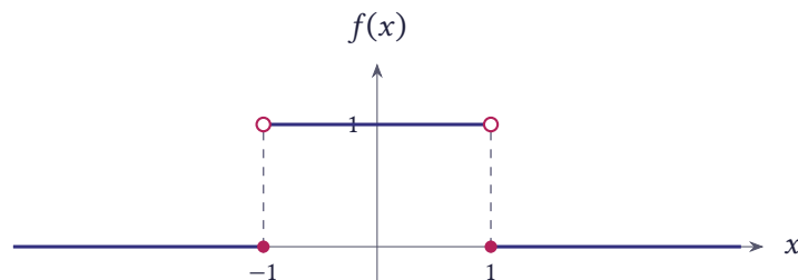
شکل ۱۰.۳ پالس مستطیلی f(x) = 1 برای |x| < 1
