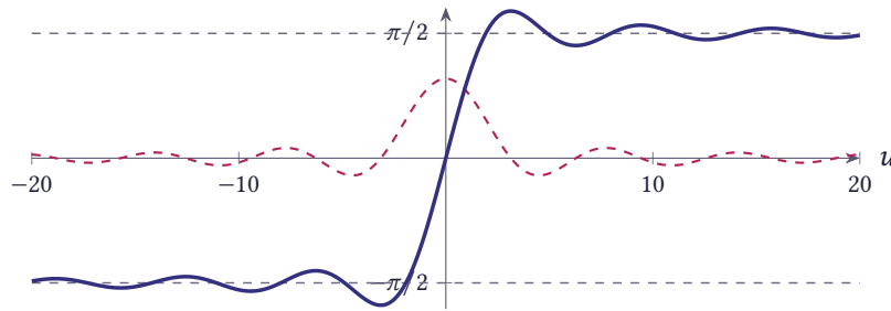
شکل ۱۰.۲ تابع \text{Si}(u) (خط ممتد) و تابع \sin u/u (خط چین)
