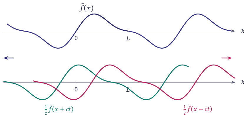
شکل ۱۱.۵ ادامه فرد و متناوب \tilde{f}(x) و دو موج \frac{1}{2}\tilde{f}(x+ct) و \frac{1}{2}\tilde{f}(x-ct) که در دو جهت مخالف حرکت می‌کنند
