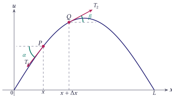
شکل ۱۱.۱ قطعه PQ از تار مرتعش: کشش‌های T_1 و T_2 در دو انتها با زوایای \alpha و \beta
