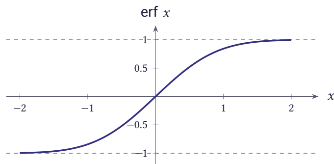
شکل ۱۲.۲ نمودار تابع خطا \operatorname{erf}(x) برای -2 \leq x \leq 2
